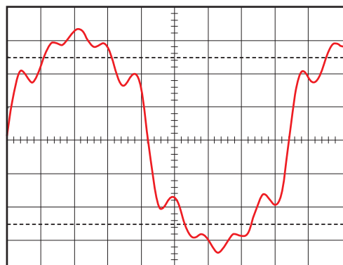
谐波波形，基波，第三，第五，第七和第九
