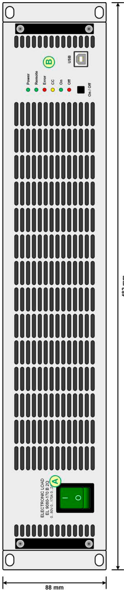
图 1 - 前视图
