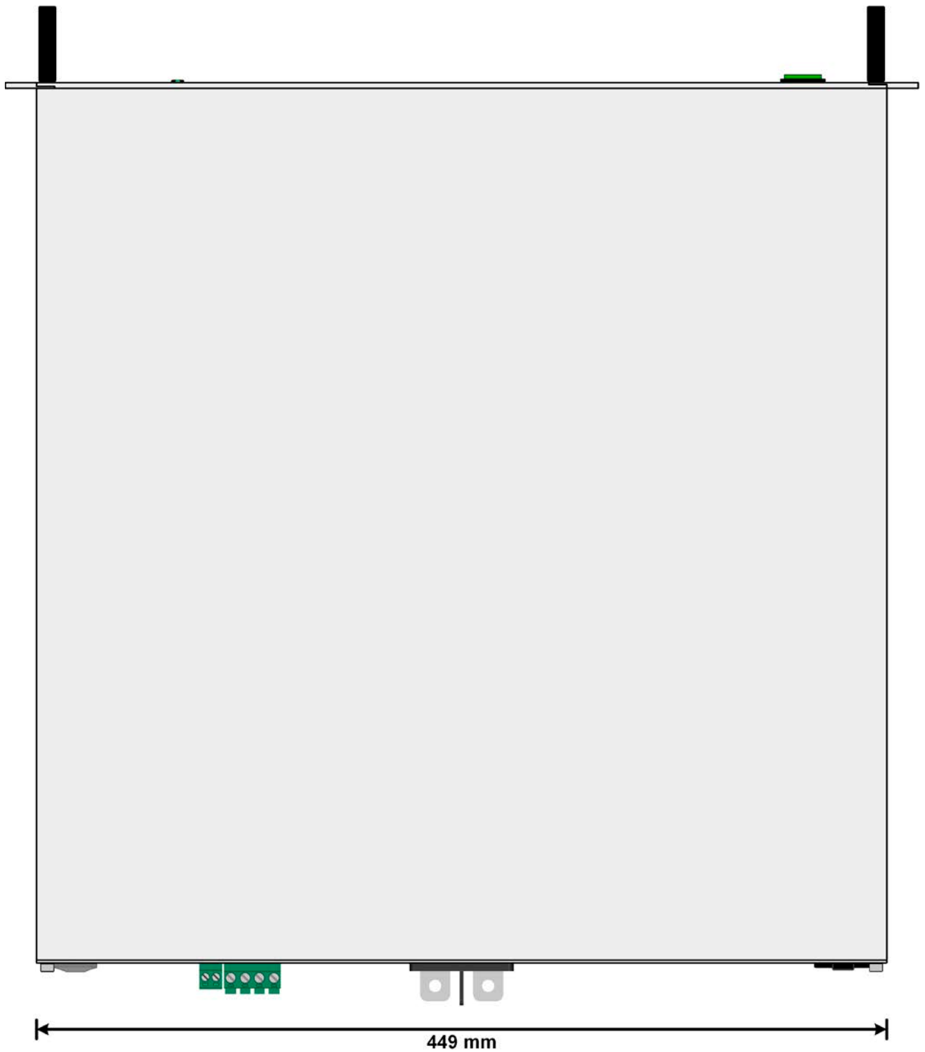
图 5 - 俯视图
