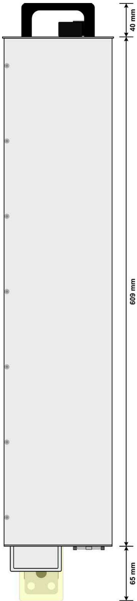
图 3 - 左侧视图
