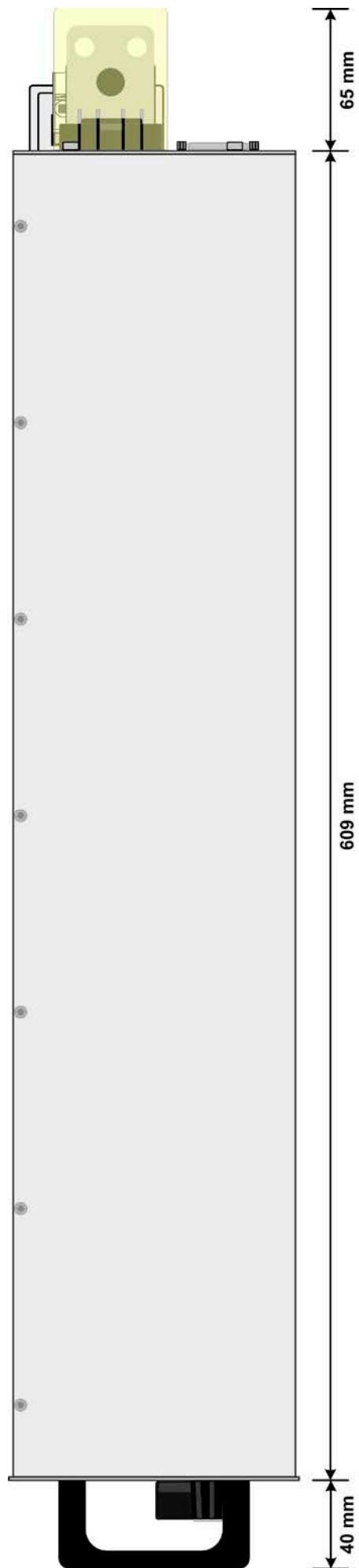
图 4 - 右侧视图
