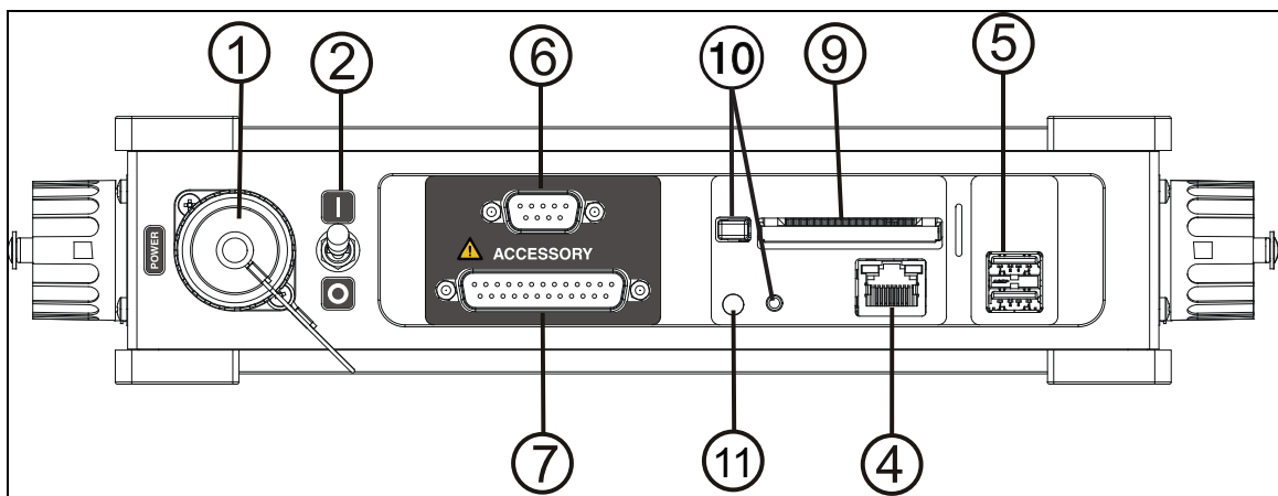
图 1-3.顶视图
