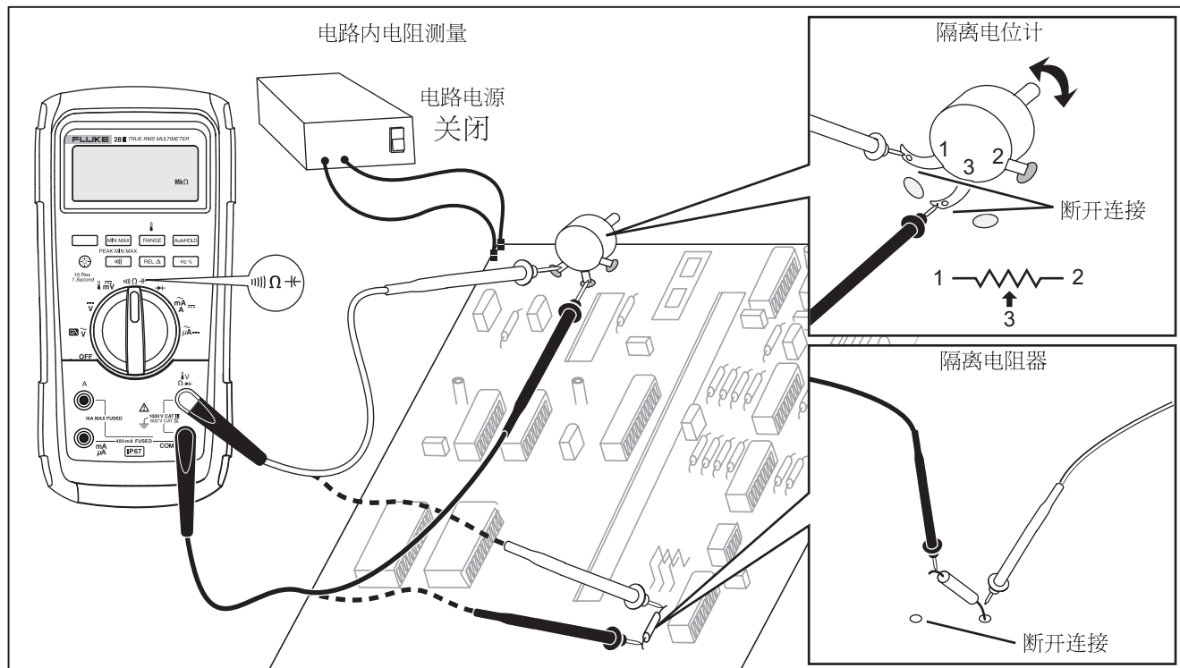
图 5.电阻测量
