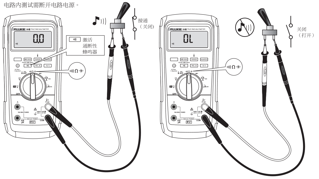
图 4.通断性测试
