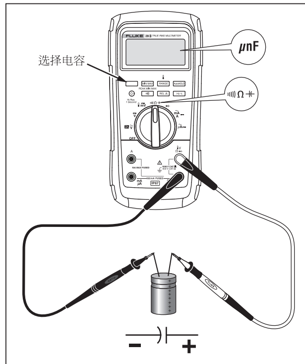
图 6. 电容测量
