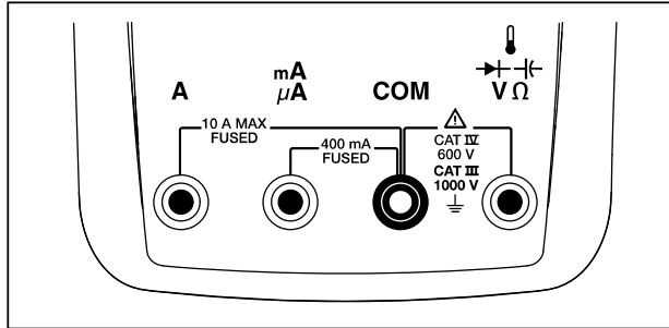
图 4.输入端子
