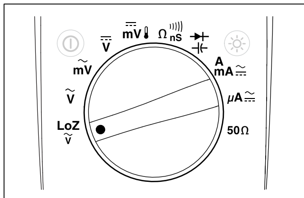
图 3. 旋转开关
