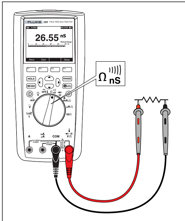
图 18. 电导测量
