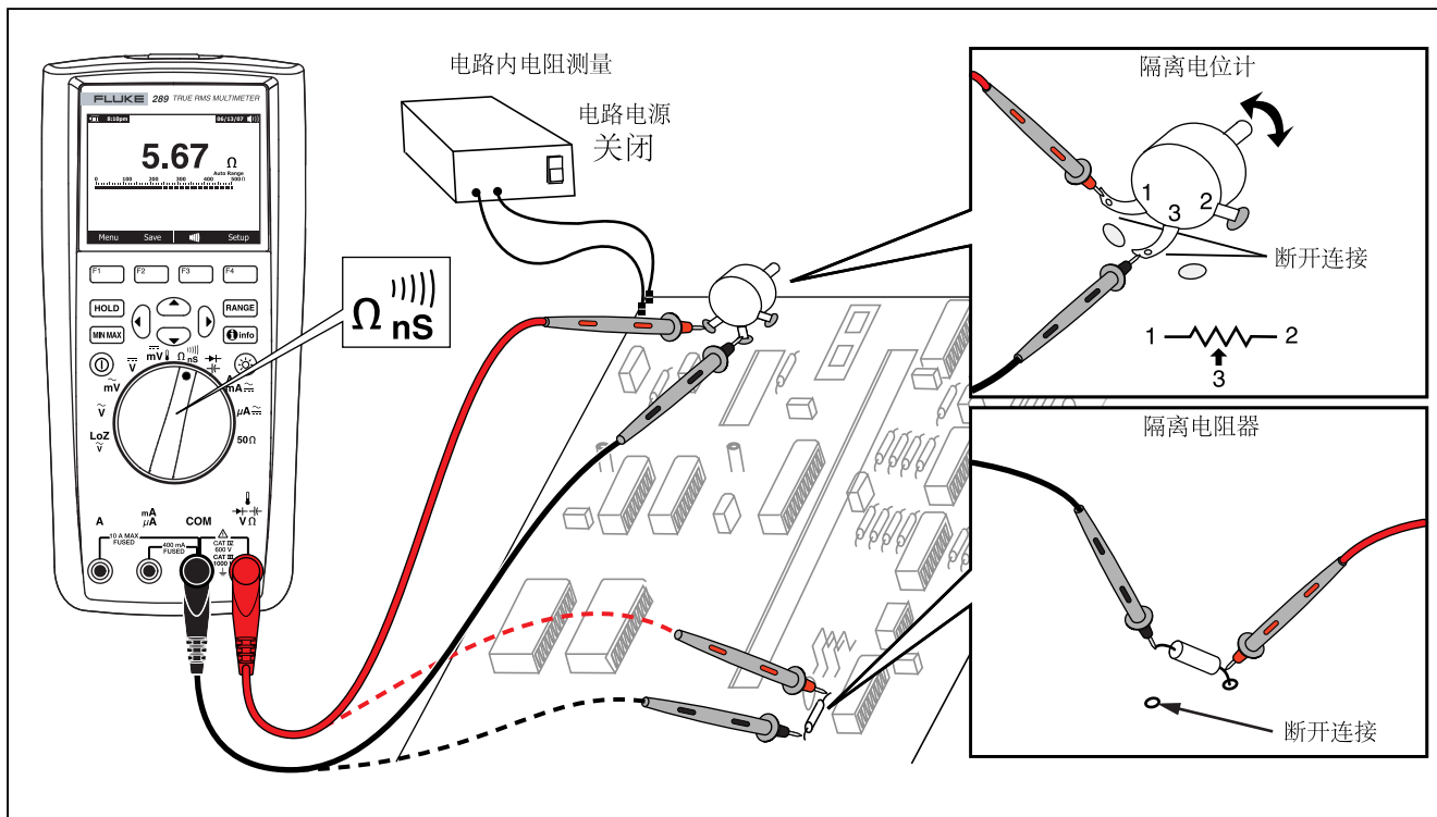
图 15.电阻测量
