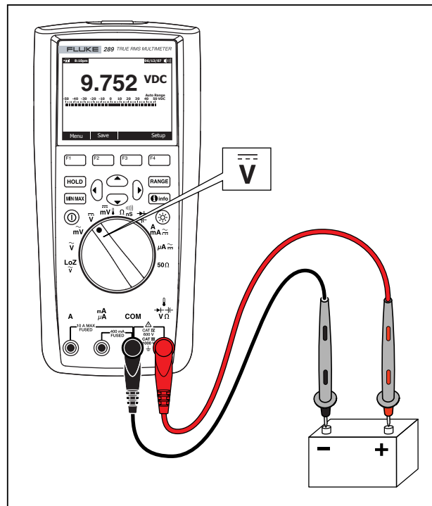
图 12.直流电压测量
