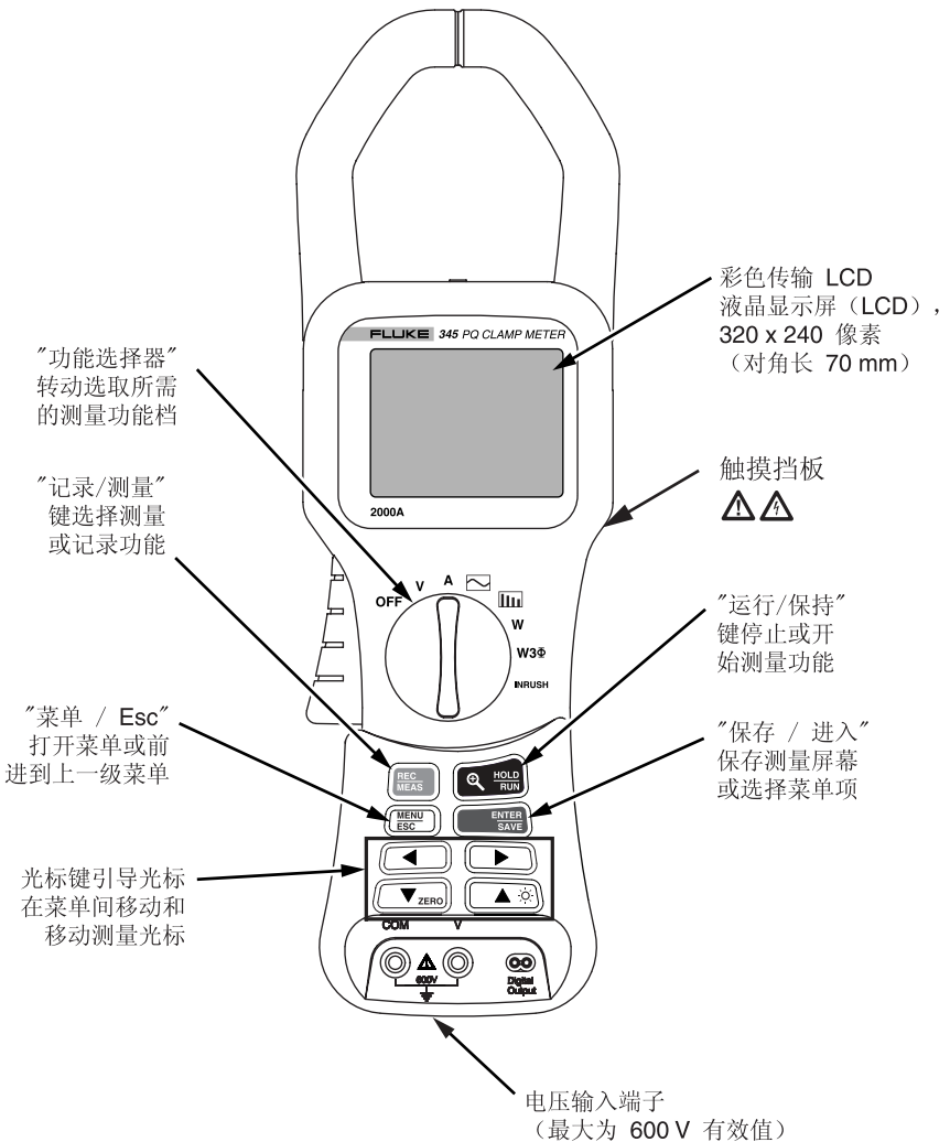
图 4. 345 正视图
