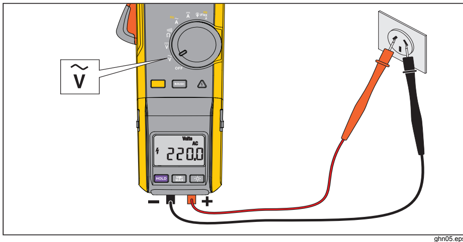
图 6. 使用测试导线测量（显示交流电压）
