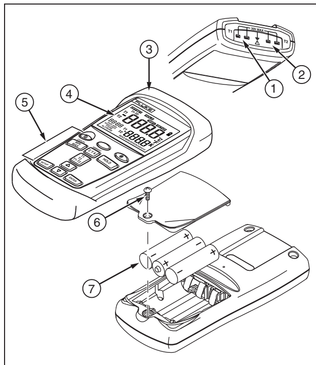
图 1. 部件
