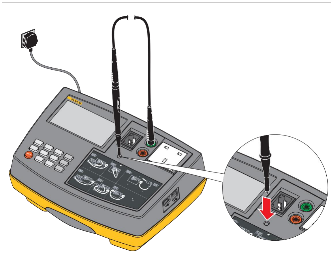
图 1 接地调零连接
