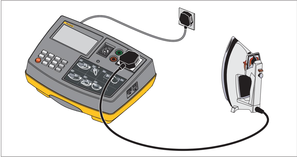
图 5 负载/漏泄电流测试连接
