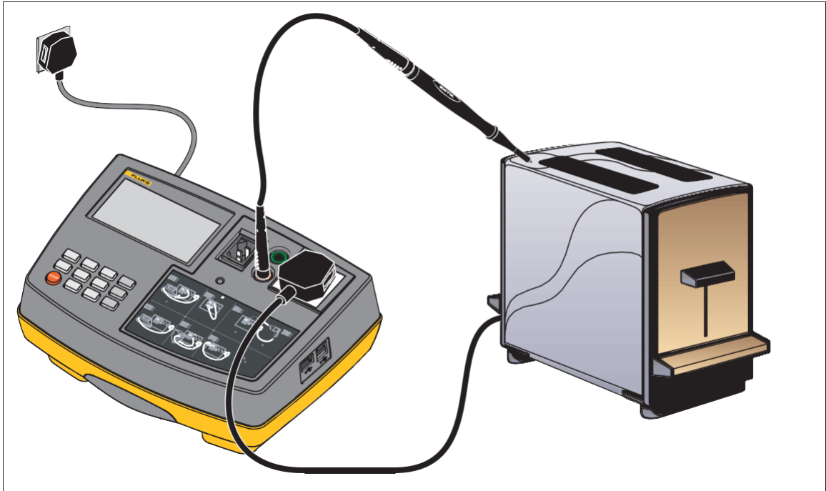
图 4 接触电流测试连接
