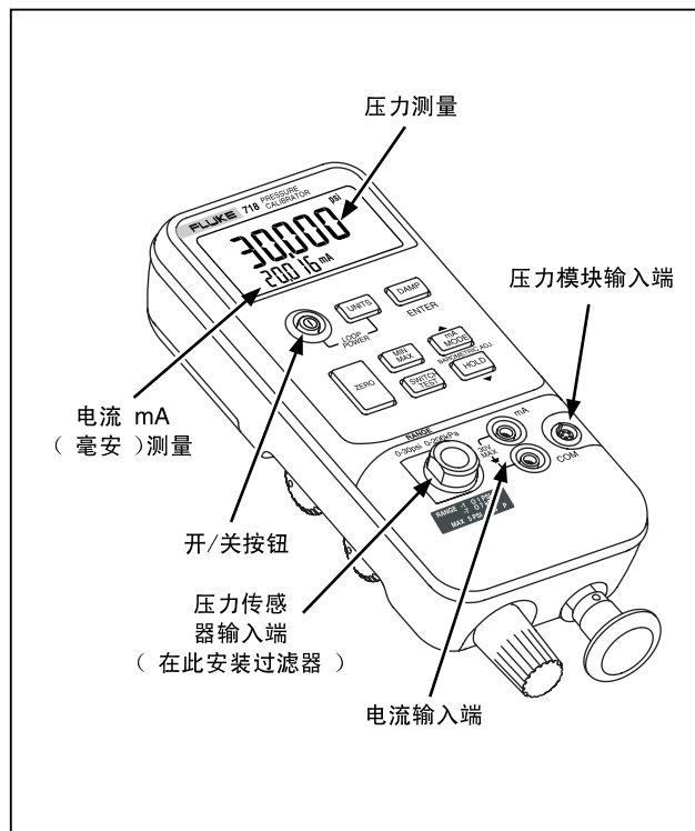
图 2. 前面板特性
