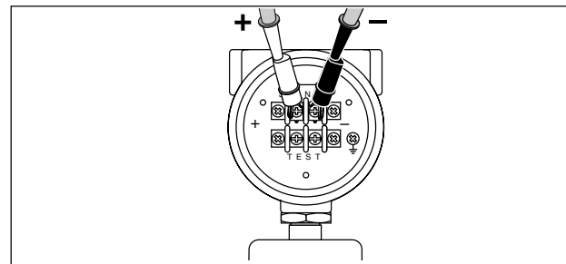
图 7. 供应回路电压
