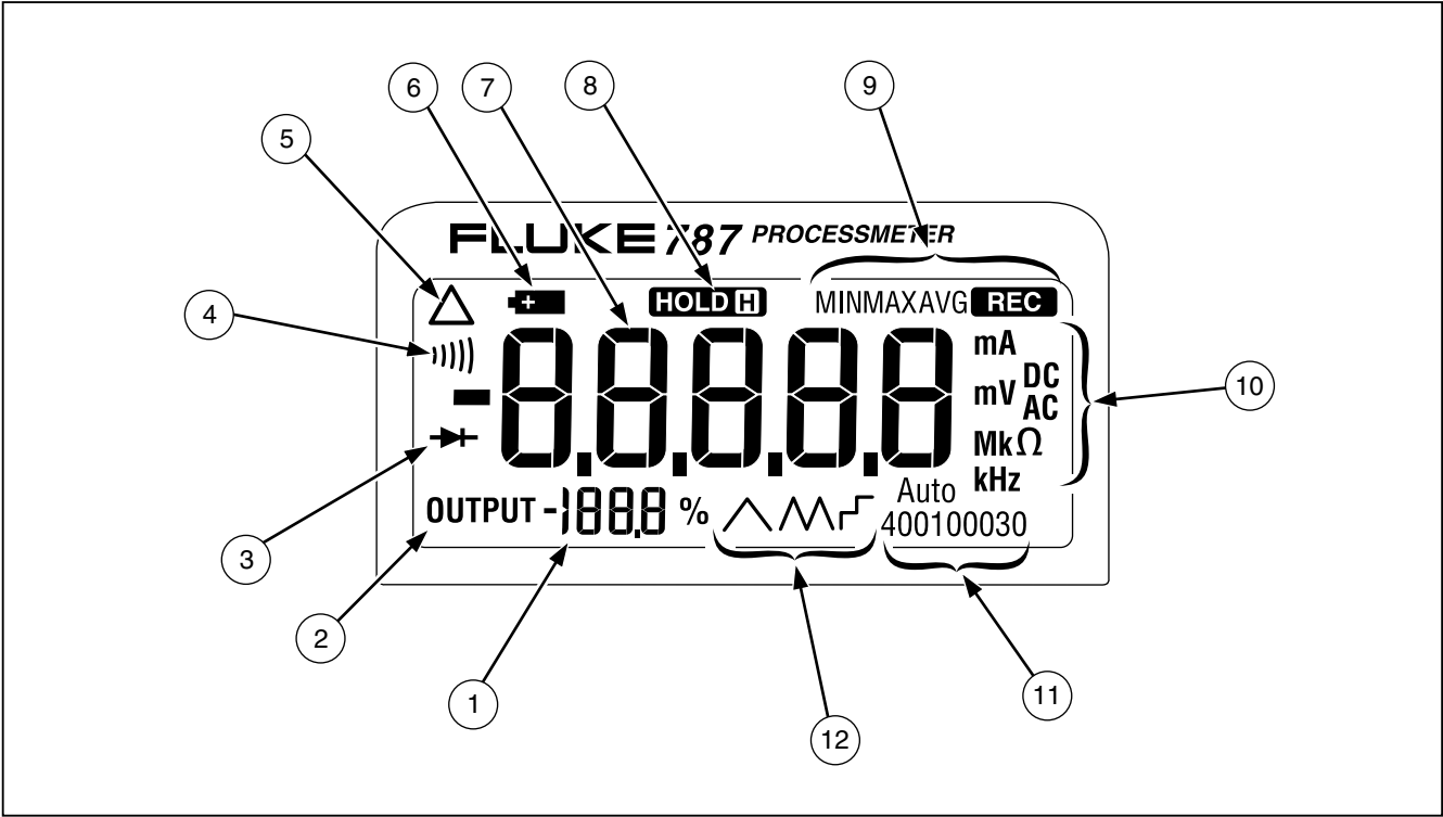
图 6. 显示的单元
