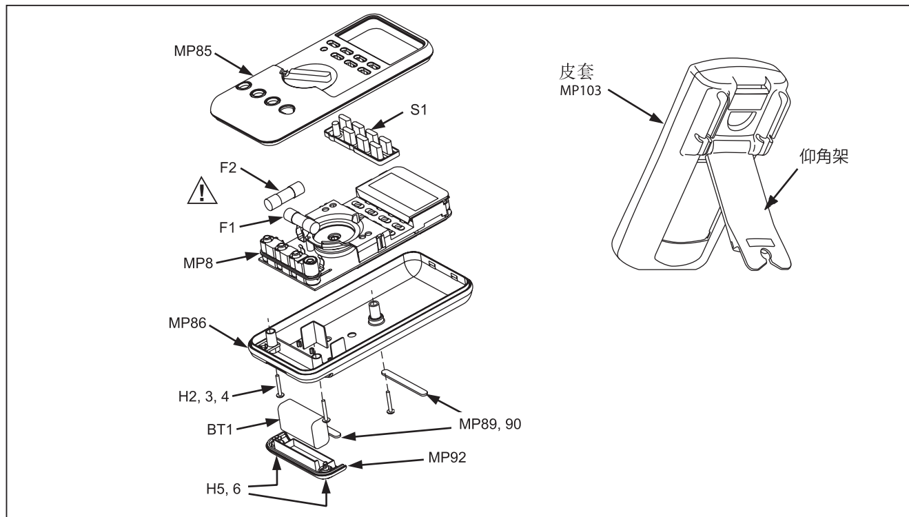
图 12. 零件
