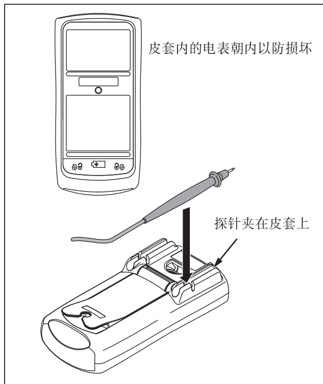
图 9. 使用皮套
