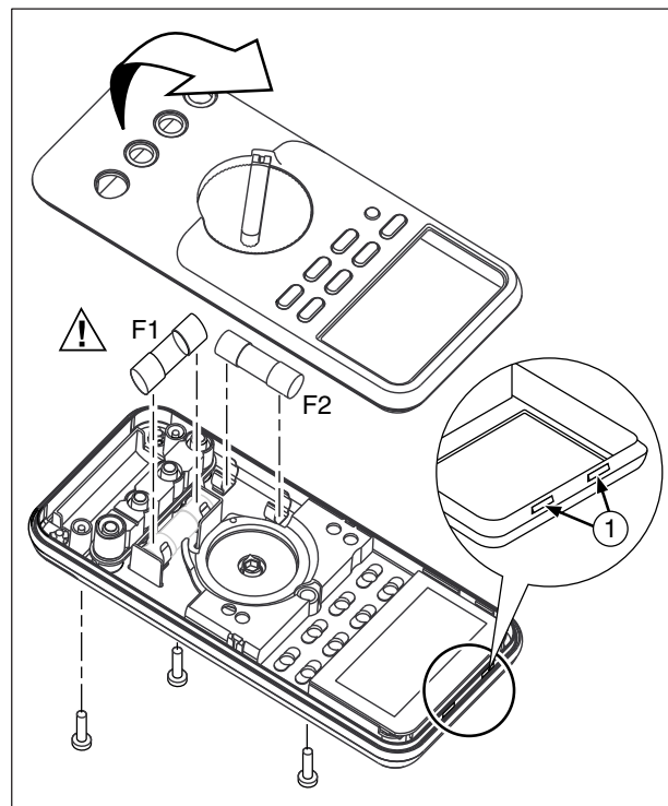
图 11. 更换保险丝
