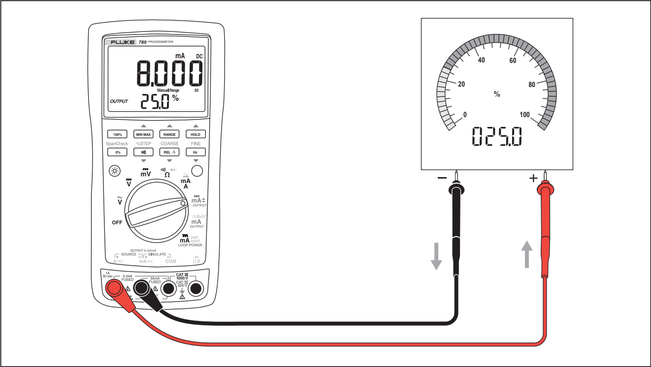
图 1.输出电流
