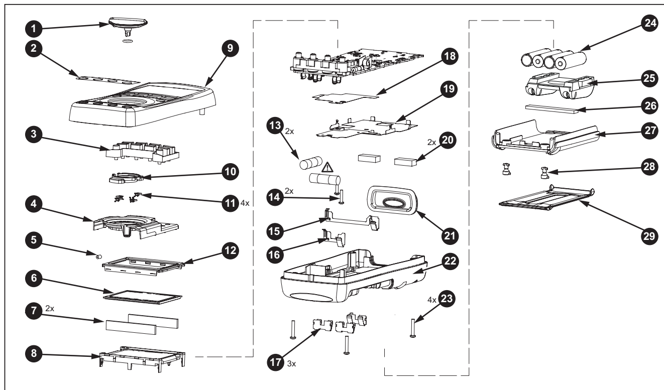
图 6. 替换零件
