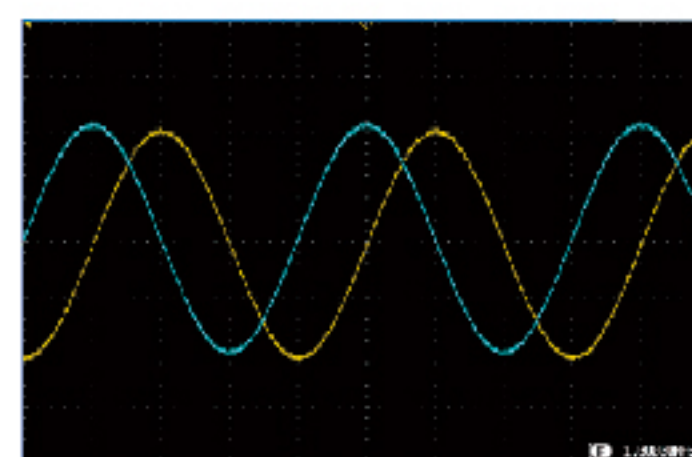
正交(正弦和余弦)信号
