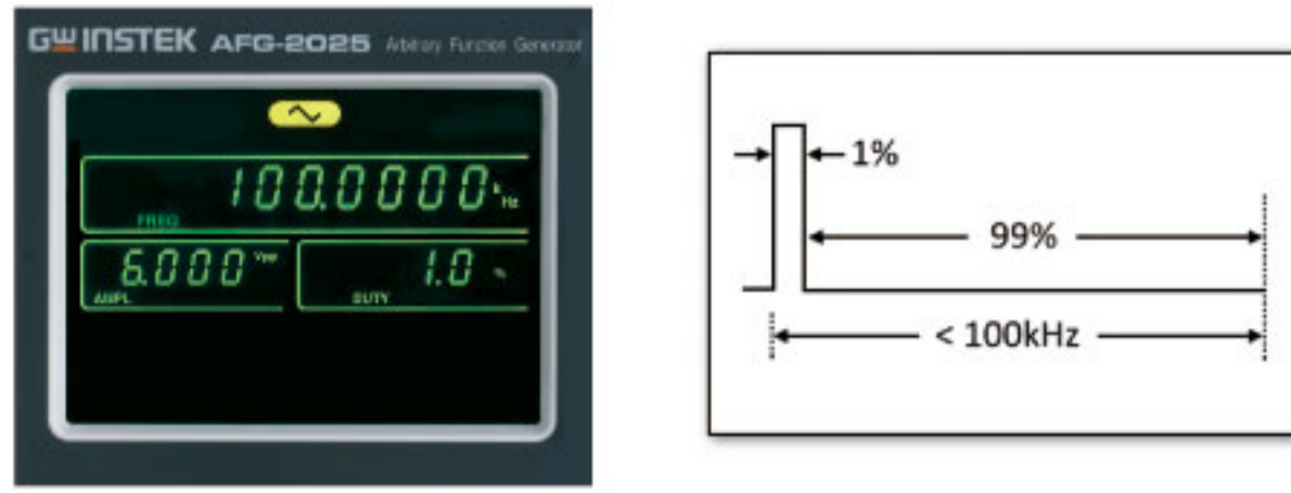
设置 1% 的方波占空比
