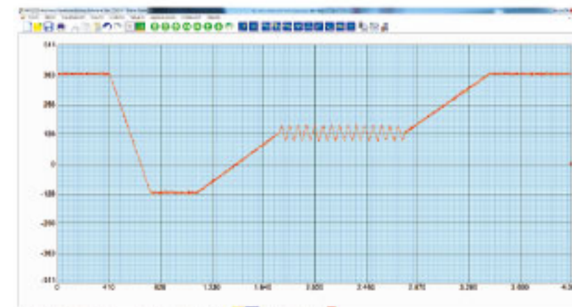
任意波形编辑 PC 软件
