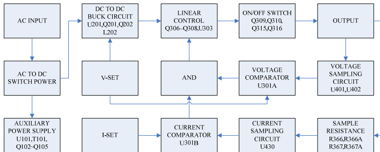
方框图
