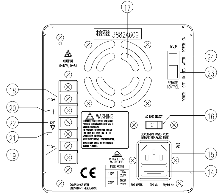
● 图 4-3 后面板
