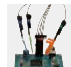
逻辑探头 连接示例
