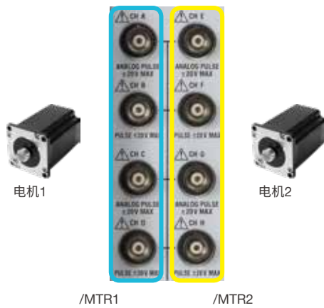
一台独立的WT5000配置用于2台电机的同时和同步测量，以确定扭矩、转速以及A/B相的方向和电角度。
