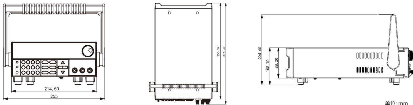
IT6722/IT6722A 机型尺寸图
