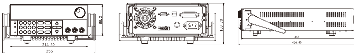
IT6723H/IT6724H/T6723G 机型尺寸图
