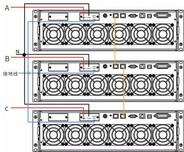
星形接法
