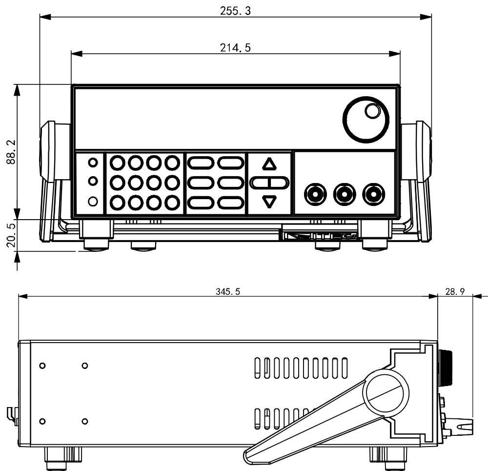
详细尺寸图
