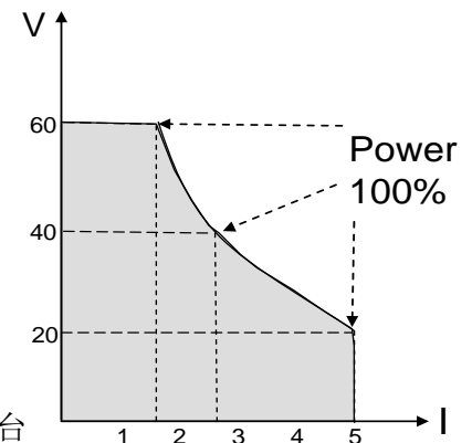
IT6922A 输出 I-V 曲线图
