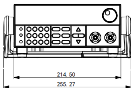
详细尺寸图
