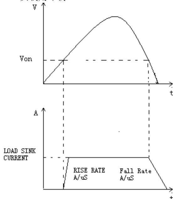
图 3-5 VON LIVING 开启时负载工作范围图
