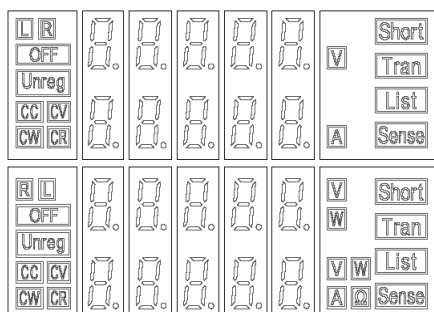
图 3-4 负载模块 VFD 面板
