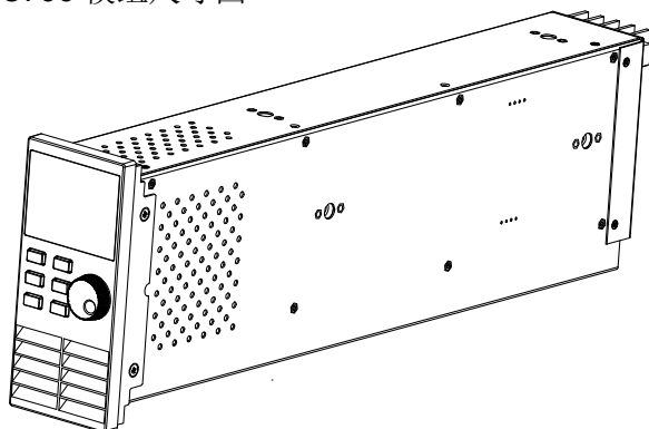
详细尺寸图
