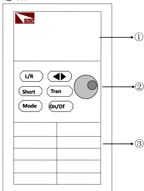
图 3-3 双路输入模组面板
