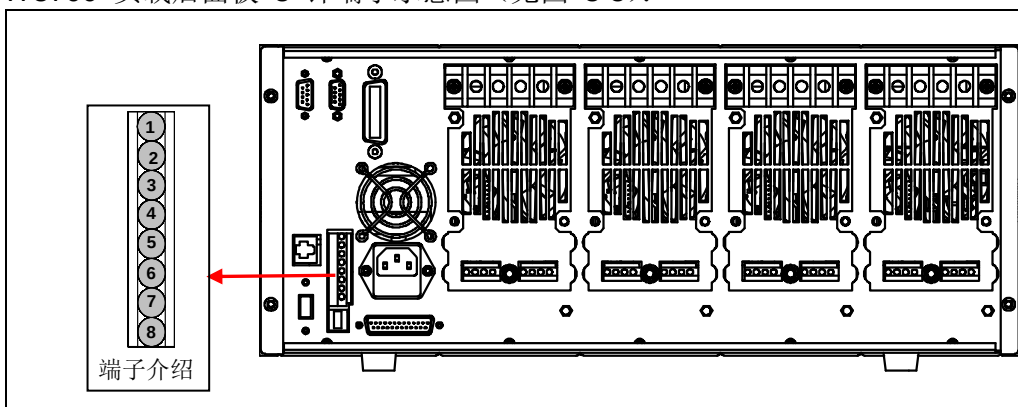
图 3-5 IT8700 后背板 8 针端子（以 IT8702 为例）
