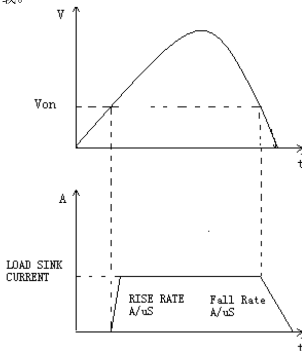
图 4-10 VON LATCH 关闭时负载工作范围
