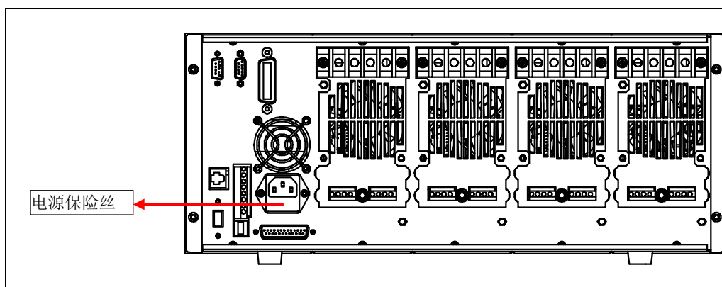
图 2-3 保险丝的位置（以 IT8702 为例）
