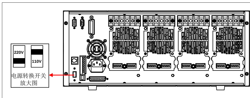
图 1-4 电源转换开关图
