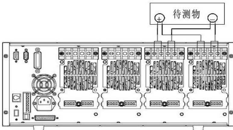
图 3-12 负载并联连接图
