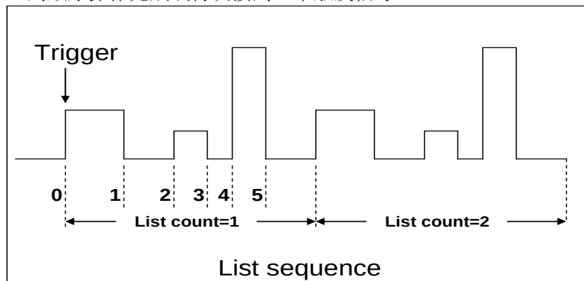
图 4-9 List 模式电流波形
