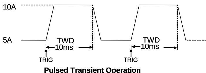
图 4-7 脉冲模式电流波形
