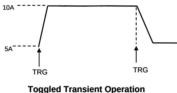
图 4-8 触发模式电流波形
