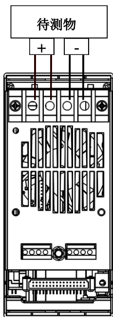
图 3-11 负载连接待测物例图
