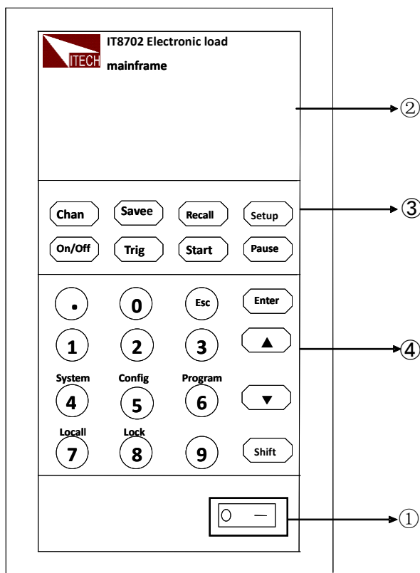
图 3-1 IT8702 主机框前面板图
