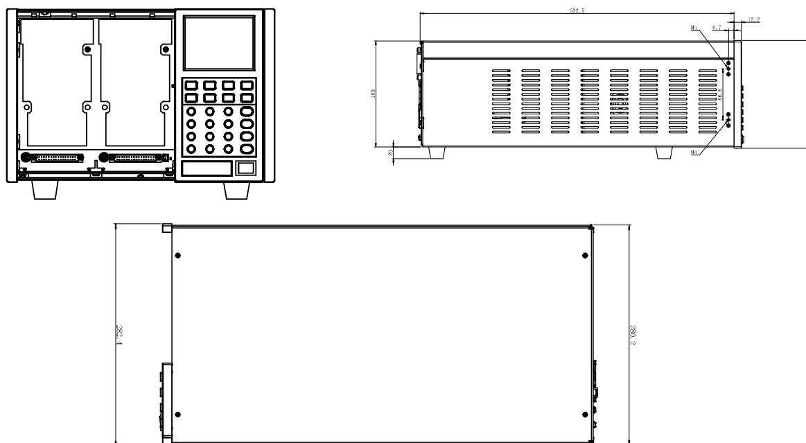
IT8701 整机安装图
