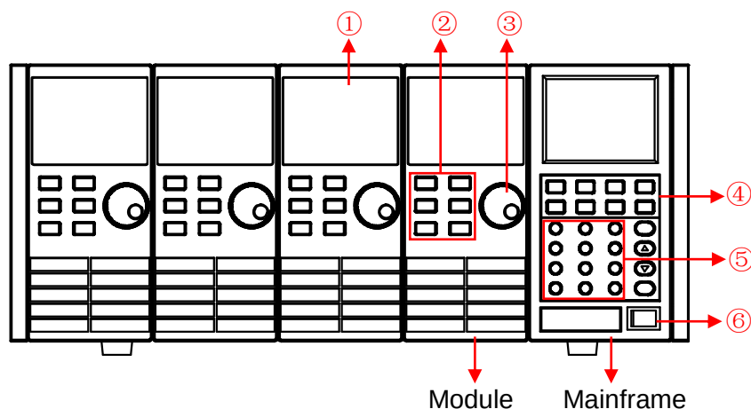
图 2-1 IT8700 前面板图（以 IT8702 为例）
