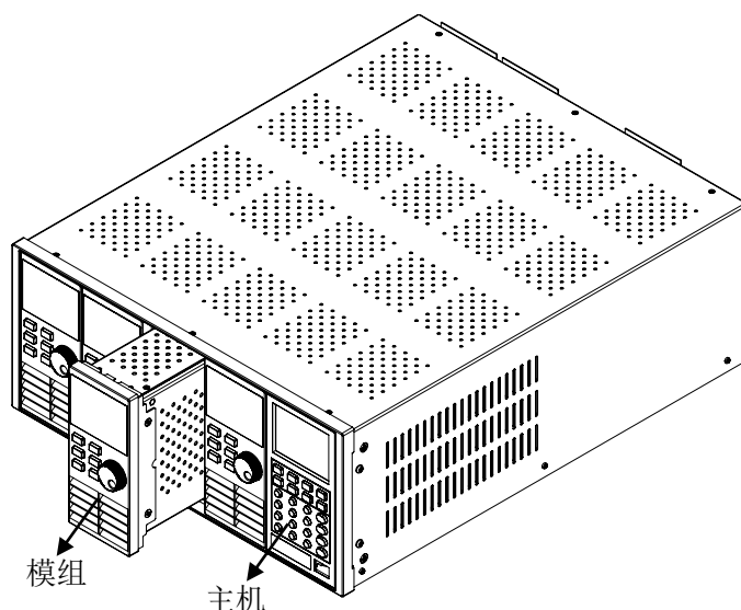
图 1-1 模组安装图
