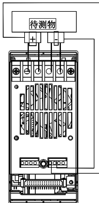
图 3-10 远端量测连接图
