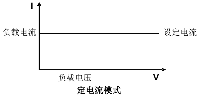
图 4-1 CC 模式电压电流关系图
