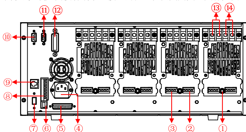
图 2-2 IT8700 后面板图（以 IT8702 为例）
