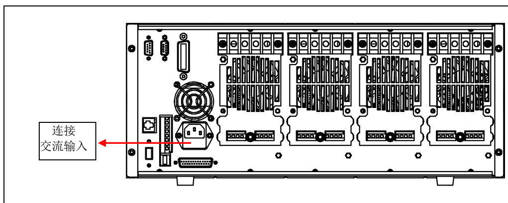
图1-5 连接交流输入图
