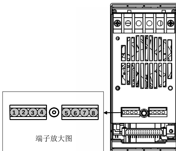
图 3-9 单路负载后面板端子功能
