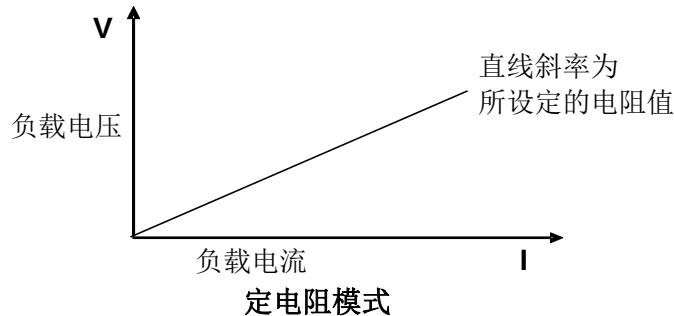
图 4-2 CR 模式电压电流关系图
