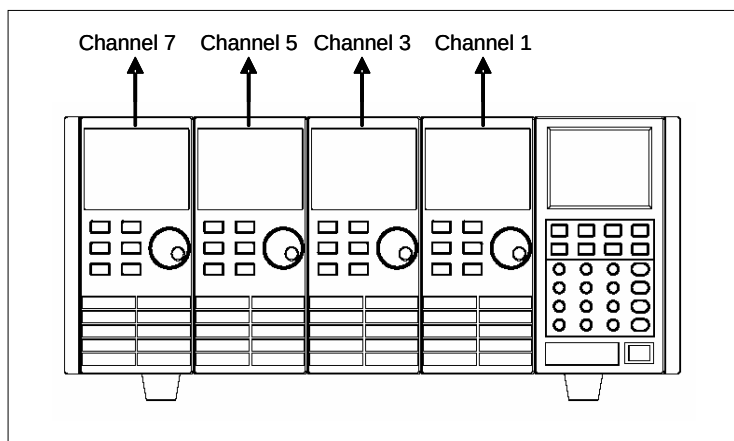
图 1-3 安装 4 个单通道模组时的通道编号分布图
