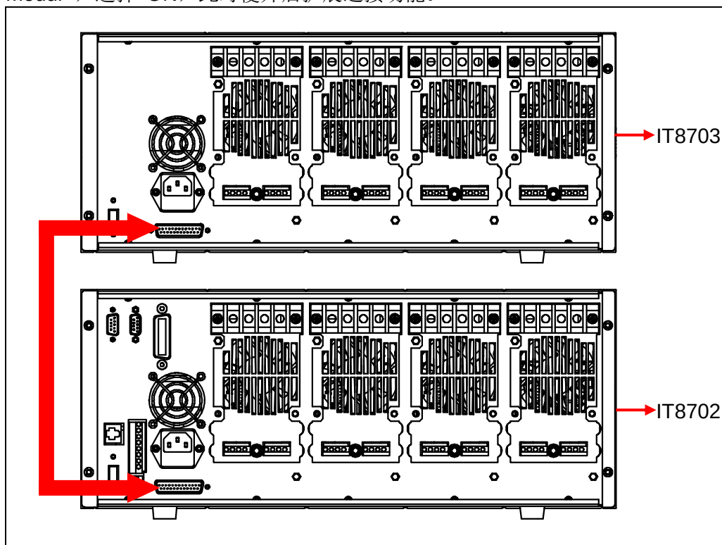
图 3-8 扩展机框连接图
