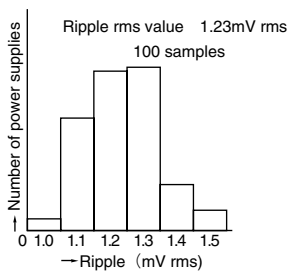
[Fig.-2 ] Ripple (Noise)
