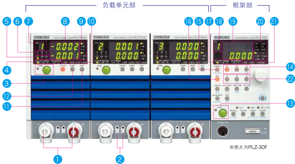
前面板
