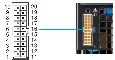
J1 连接器的端子排列
