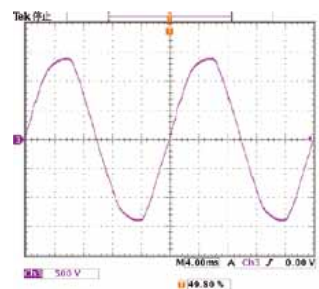
▲ 转换变压器方式的 AC 输出波形
