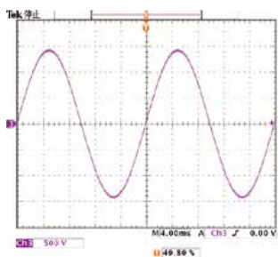
▲ TOS5300 系列的 AC 输出波形
