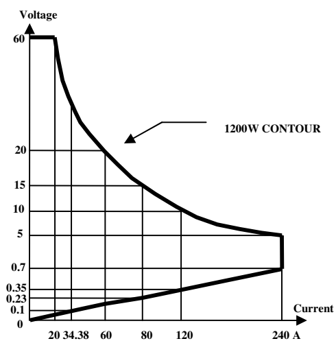
圖 1-3 3352F 高功率電子負載功率曲線圖
