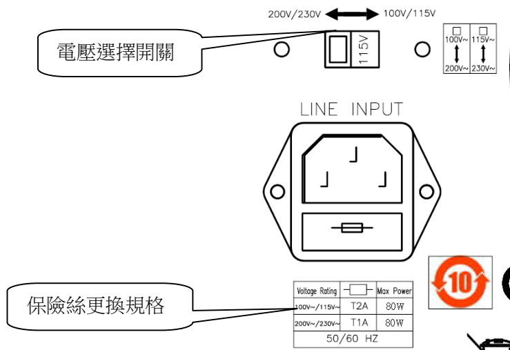
圖 2-1 電源設定圖
