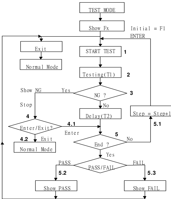
圖 3-10 測試模式操作流程圖
