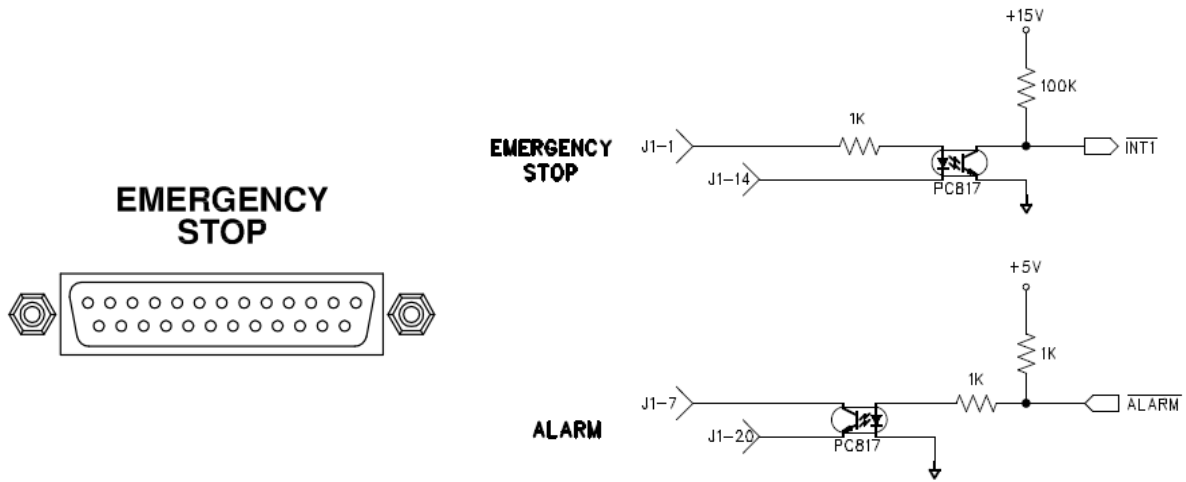
圖 2-9 緊急開關聯接器
