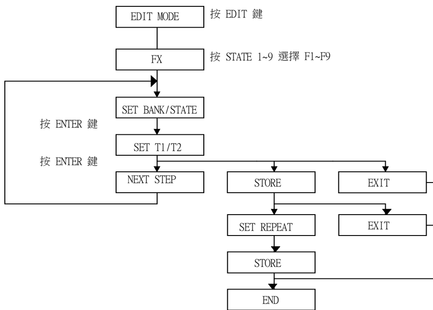
圖 3-9 編輯模式操作流程圖
