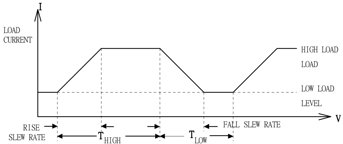
圖 1-11 動態負載電流波形圖
