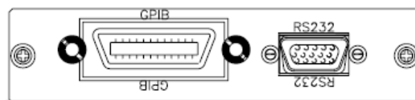
圖 2-7 3350F 系列 RS-232 + GPIB 連接埠圖
