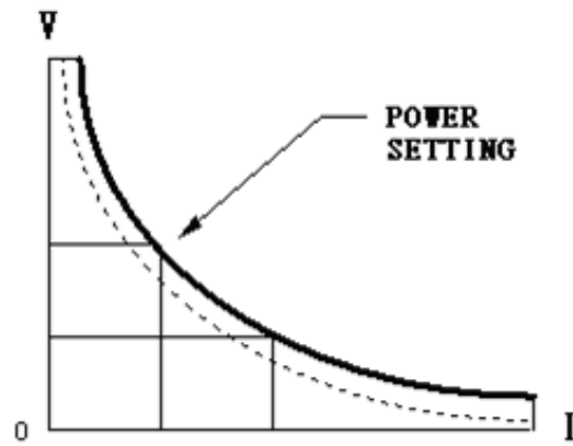
圖 1-10 固定功率模式特性圖
