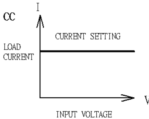
圖 1-7 固定電流模式特性圖
