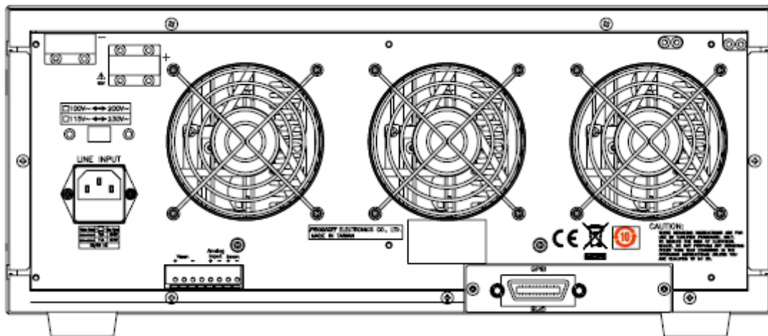
圖 2-3 3350F GPIB 連接埠圖
