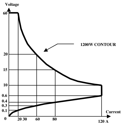
圖 1-1 3350F 高功率電子負載功率曲線圖
