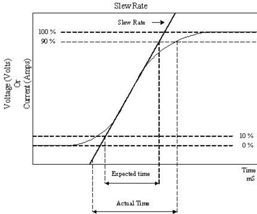
圖 1-11 回轉率(Slew Rate)曲線圖
