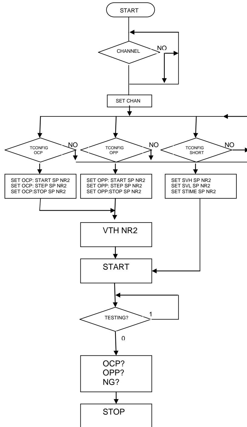
圖 4-11 3310F 系列電子負載OCP、OPP、SHORT操作流程圖
