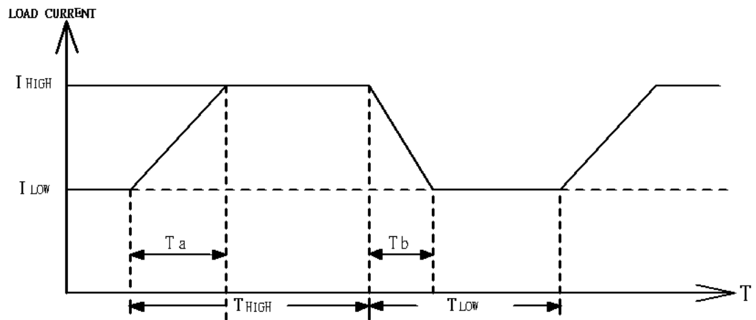
圖 4-4 動態負載電流
