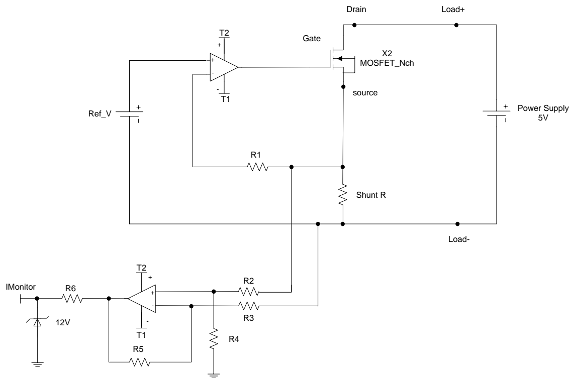
圖 3-3 3310F系列 I-monitor 等效電路圖
