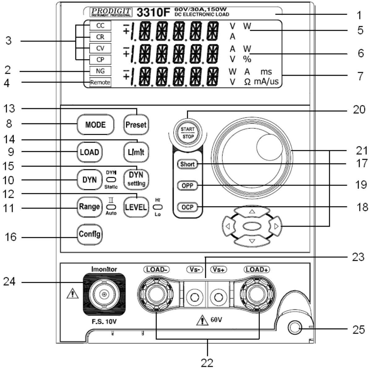
圖 3-1 前面板圖
