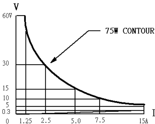
圖 1-5 3315F 0-60V/0-15A 75W 電子負載功率曲線圖
