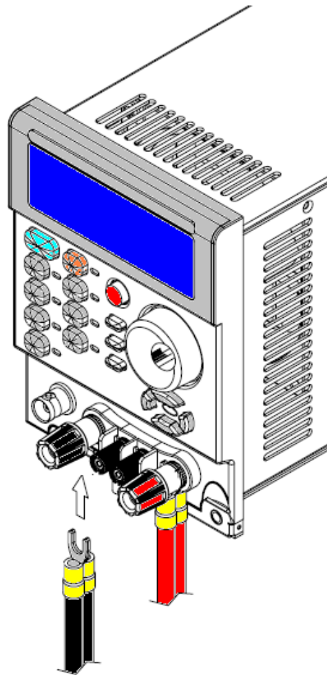
圖 3-7 Y型端子連接圖
