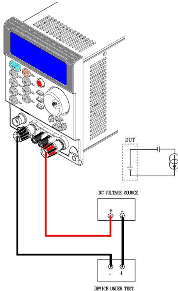
圖 4-10 高功率電子負載最低工作電壓為 0V 時的連接圖
