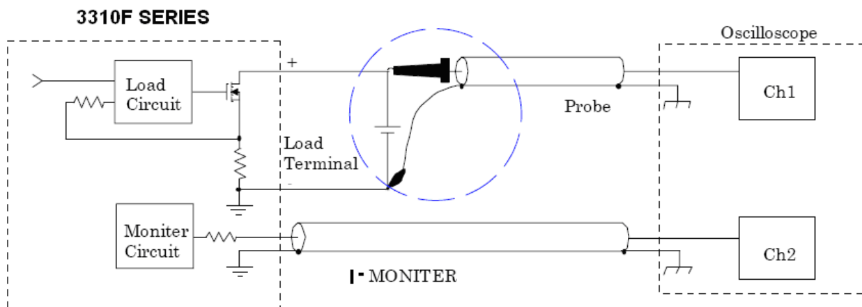
圖 3-4 示波器正確的連接圖
