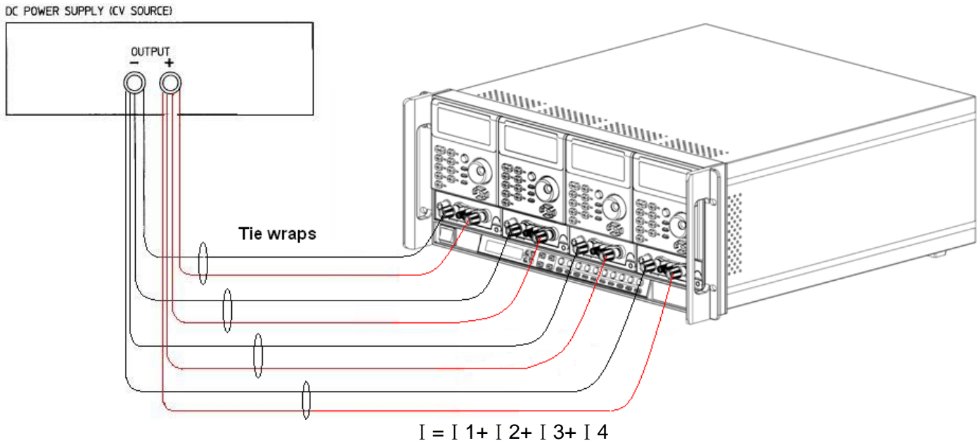
圖 4-9 電子負載多組並聯之連接圖
