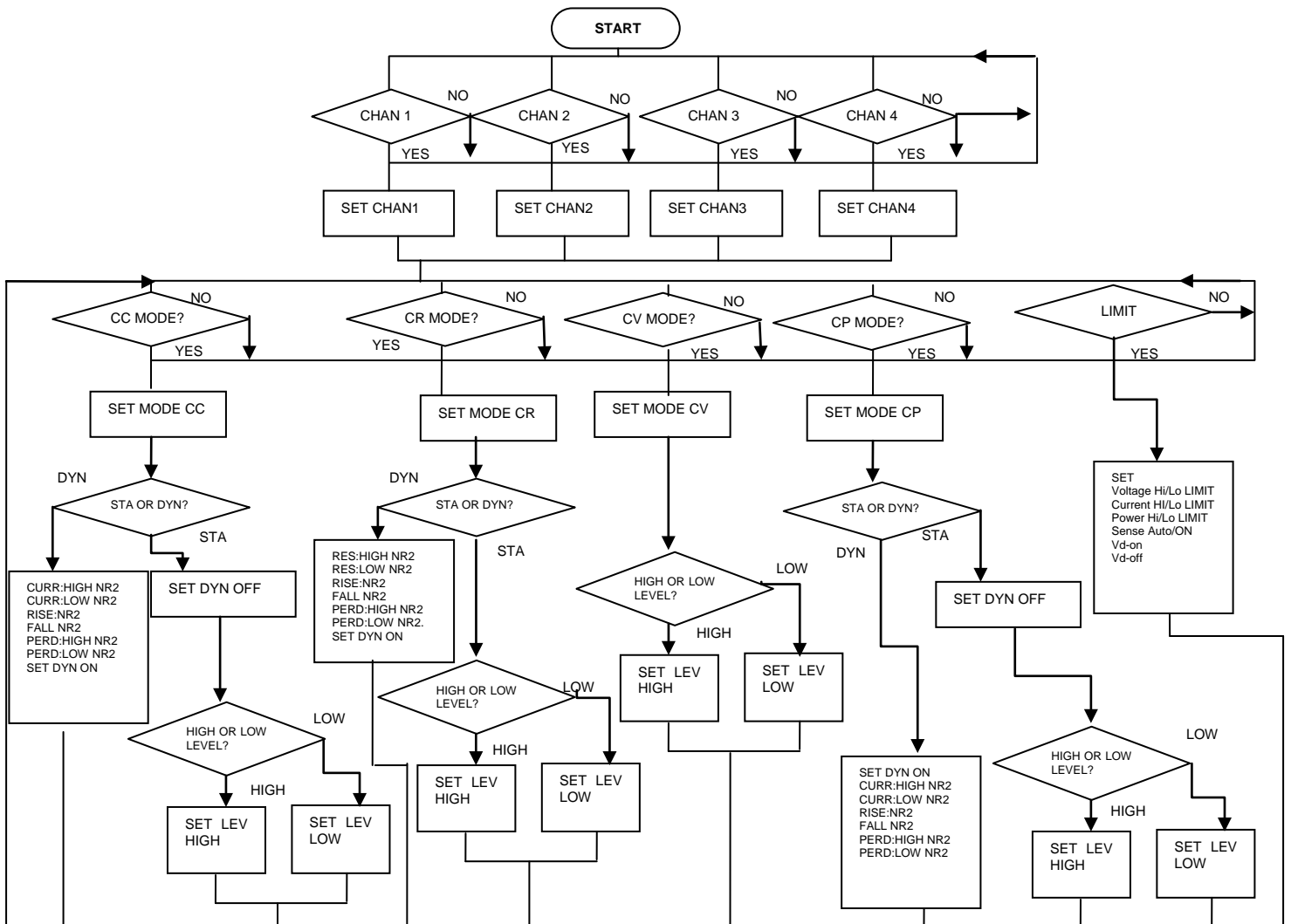
圖 2-3 3310F 系列電子負載操作流程圖
