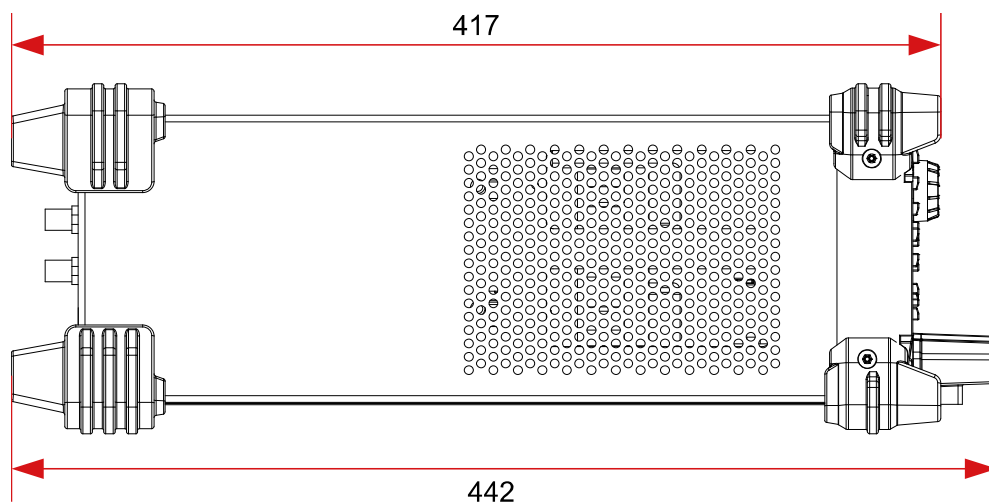
图 1-2 侧视图
