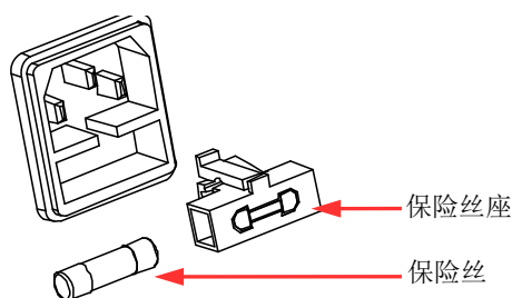
图 1-7 更换保险丝
