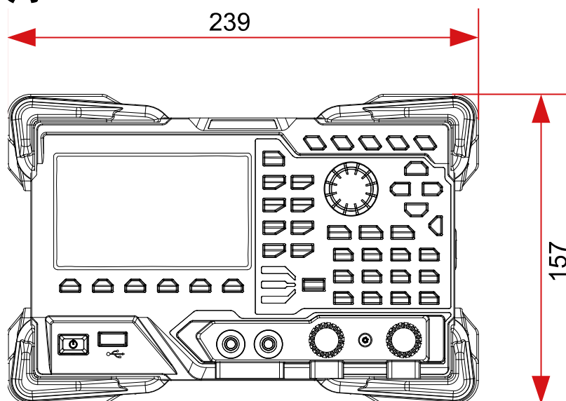
图 1-1 正视图
