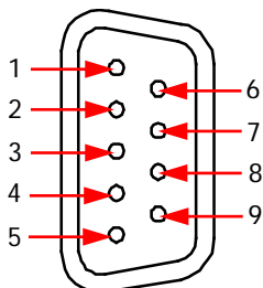
图 2-55 RS232 接口
