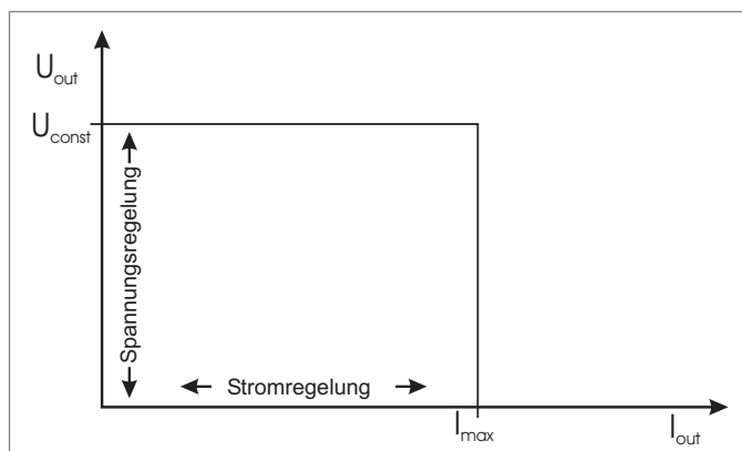
Abb. 3.7: Strombegrenzung
