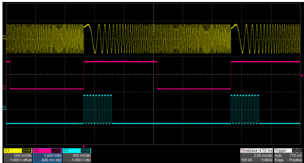
扫频和脉冲串 扫频支持“线性”和“对数”两种扫频方式，脉冲串支持“N 循环”和“门控”两种 Burst 方式。扫频和脉冲串都支持“内部”、“外部”和“手动”3 种触发源
