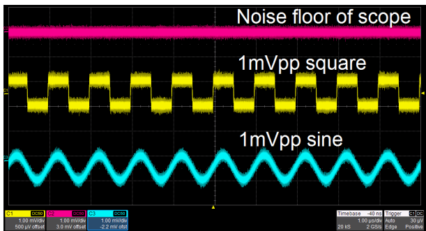
小信号 超低噪底，输出信号具有更好的信噪比
