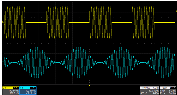
调制 支持 AM, FM, PM, FSK, ASK, PSK, DSB-AM 和 PWM 等多种模拟和数字调制方式，“内部”和“外部”两种调制信号源
