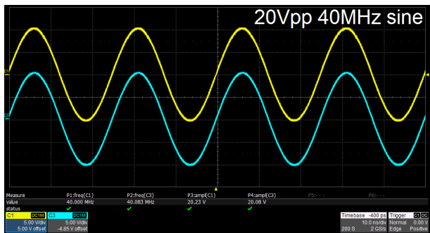
大信号 高频下的大幅度输出能力：在 40MHz 频率下仍然能保证双通道 20Vpp 满幅度输出
