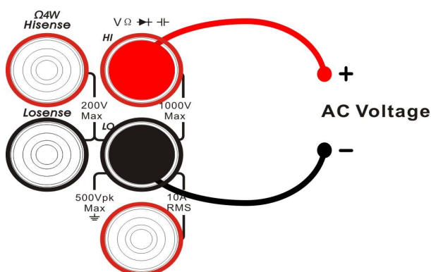
图 2-9 交流电压测量连接示意图
