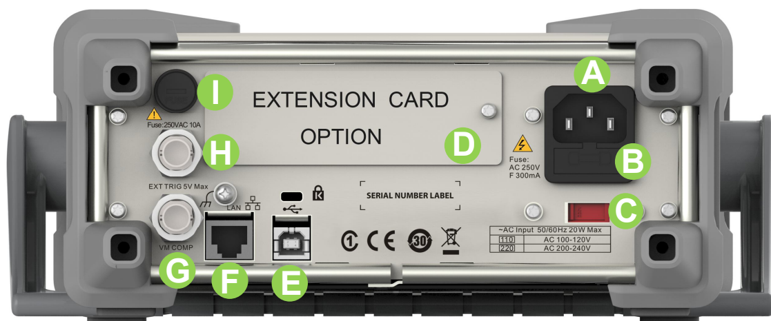
图 1-5 后面板示意图
