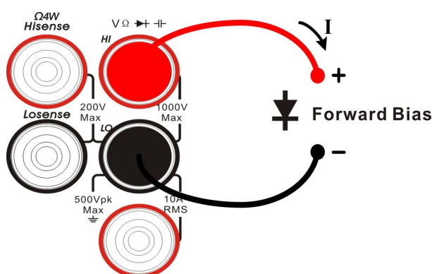
图 2-26 二极管检测示意图
