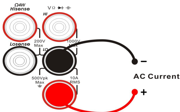
图 2-12 交流电流测量连接示意图
