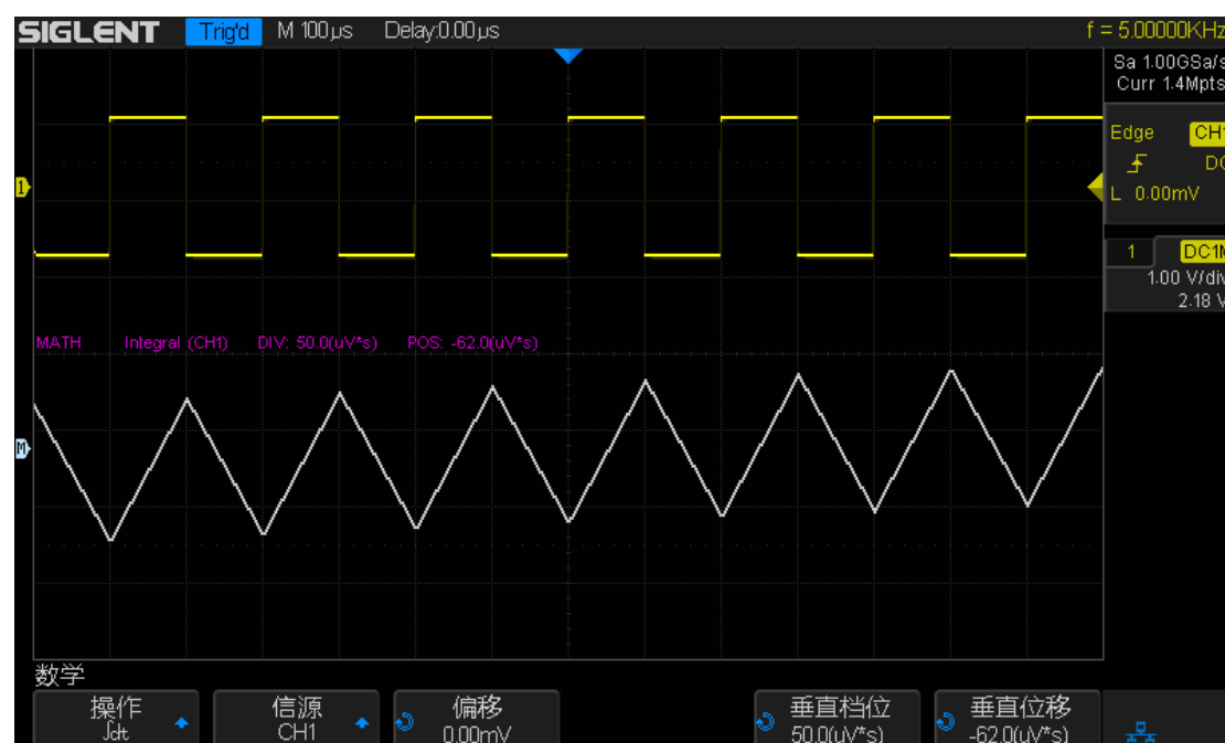
图 86 无 DC 偏移校正（积分运算）
