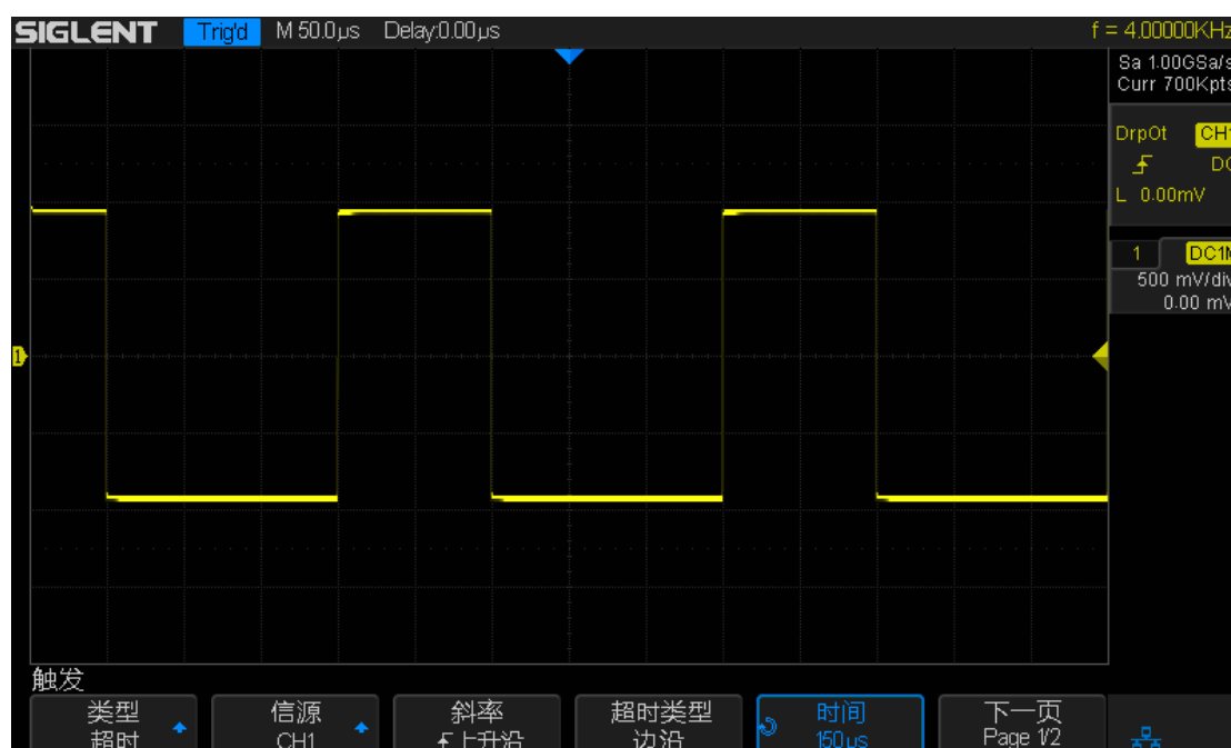
图 41 “边沿”超时触发
