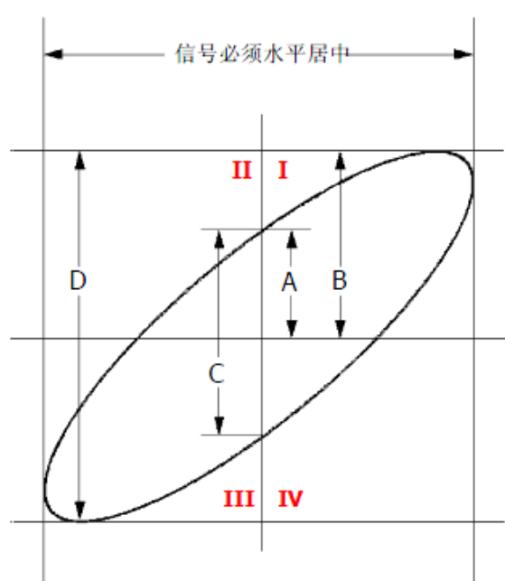
图 16 李沙育测量原理图
