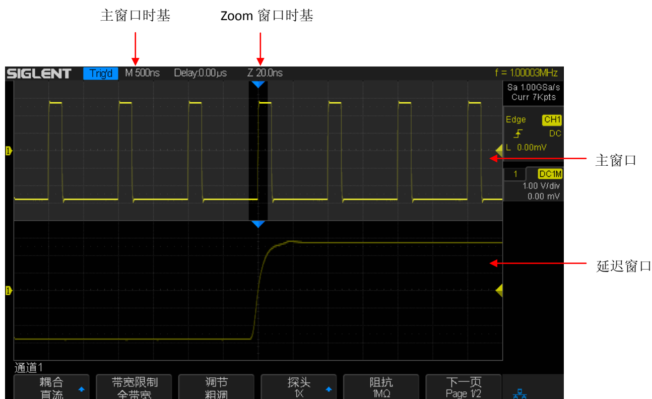
图 18 分屏缩放
