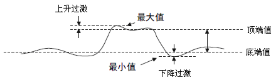
图 93 上升/下降过激示例图
