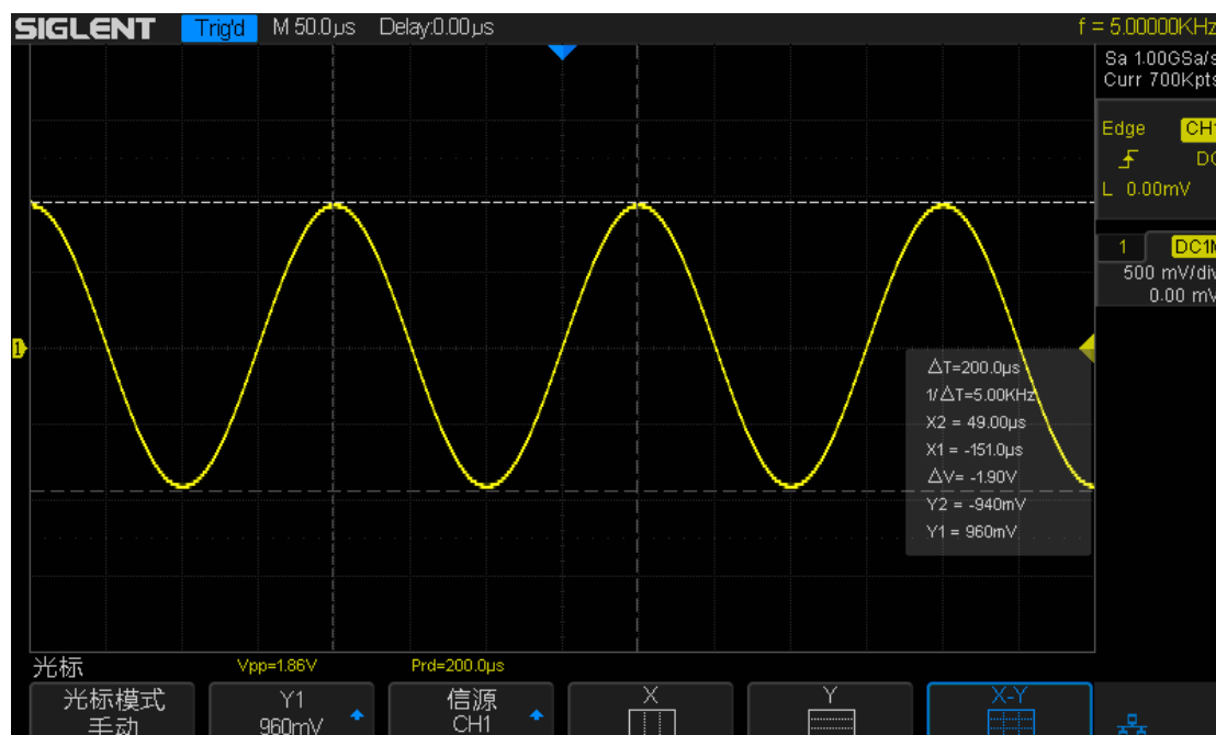
图 89 光标测量
