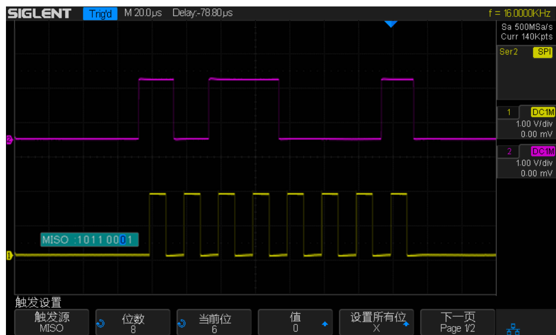
图 57 SPI 触发图
