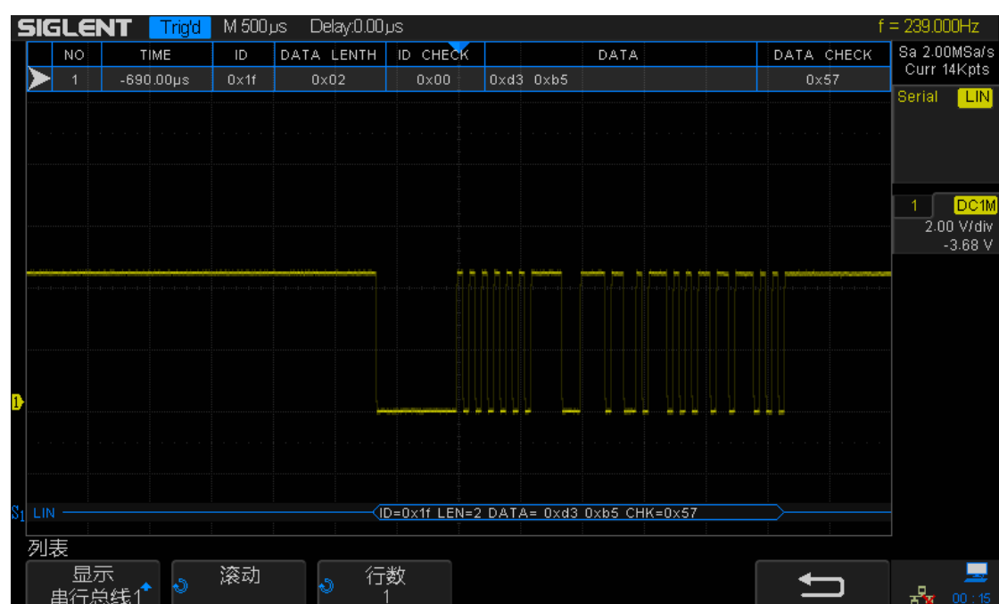
图 72 LIN 解码
