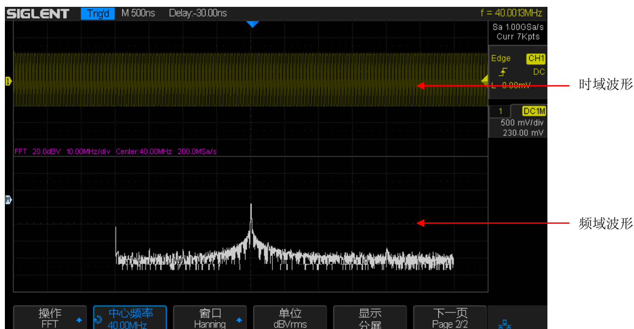
图 84 FFT 波形
