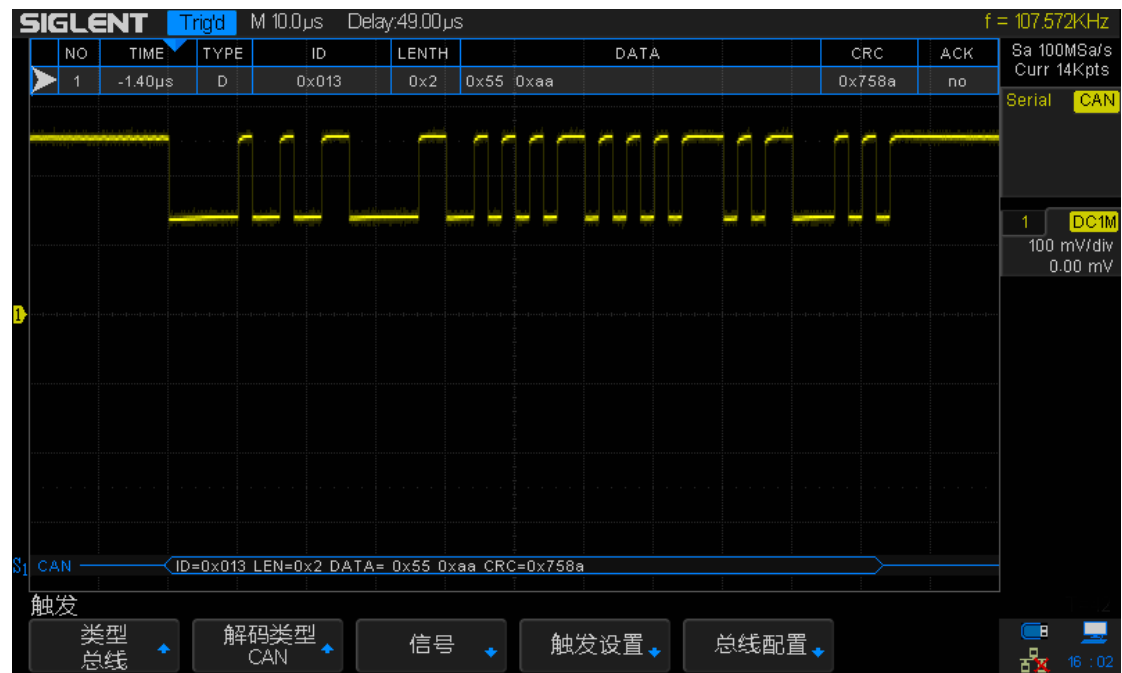
图 67 CAN 触发
