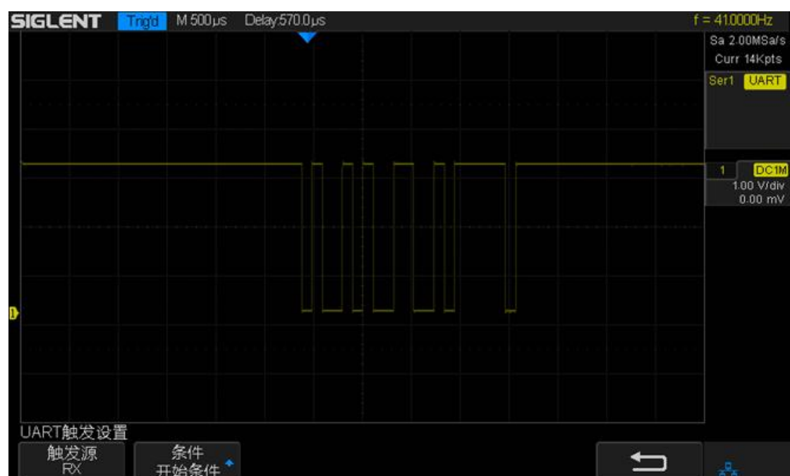
图 64 UART 触发
