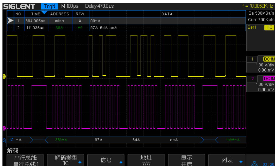
图 50 IIC 解码图
