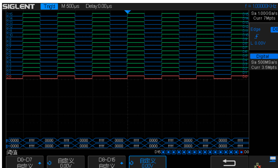
图 79 数字总线
