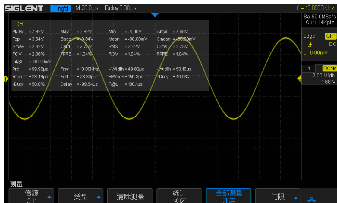
图 98 全部测量
