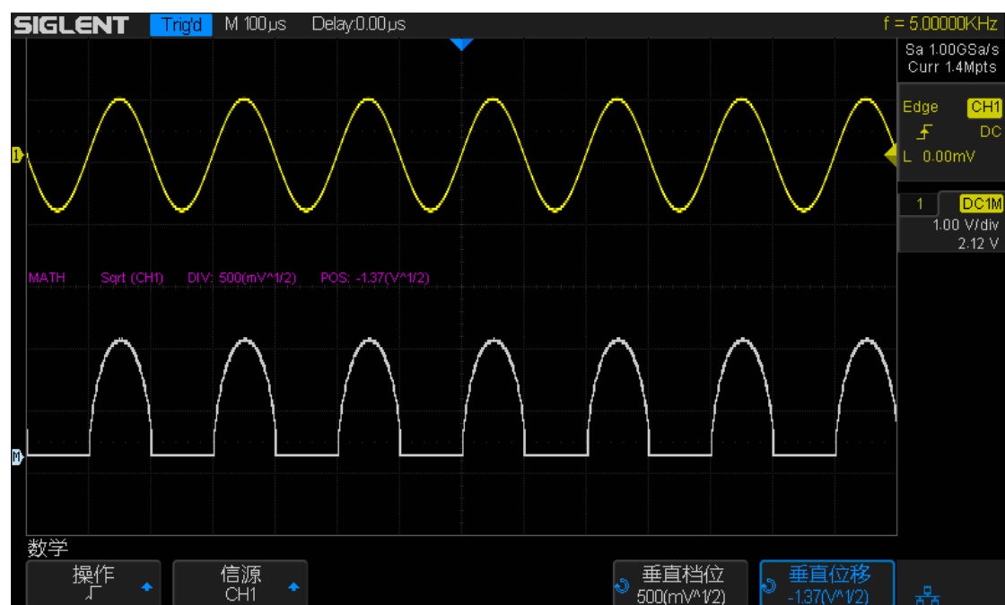
图 88 平方根运算
