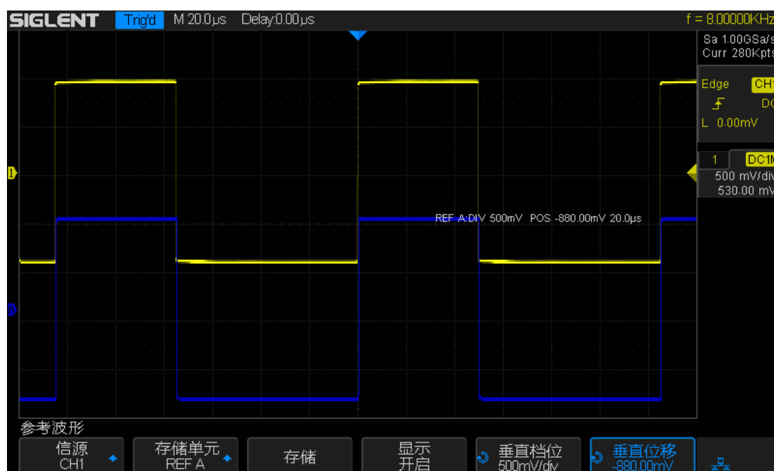
图 80 调节参考波形
