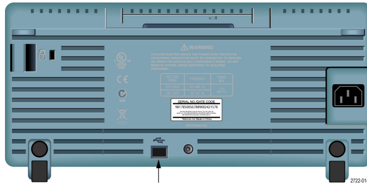
USB 设备端口
