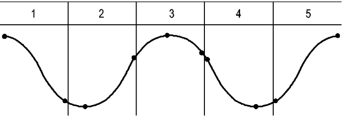
峰值检测采集间隔（1250）
