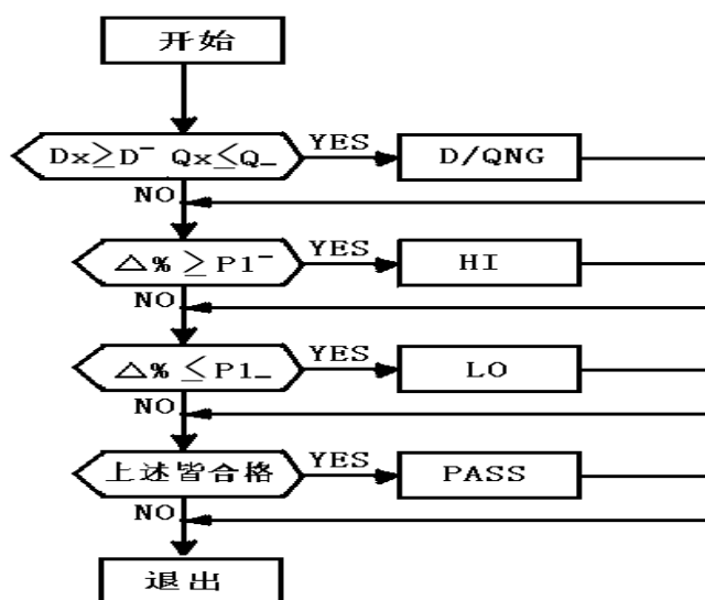
图 2-8 P1 状态的分选判别流程
