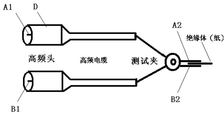
图 3-5 测试电缆局部连线图
