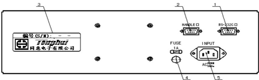
图 1-1 仪器后面板示意图
