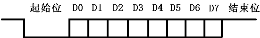
图 2-5 RS232C 串行口数据传输格式图
