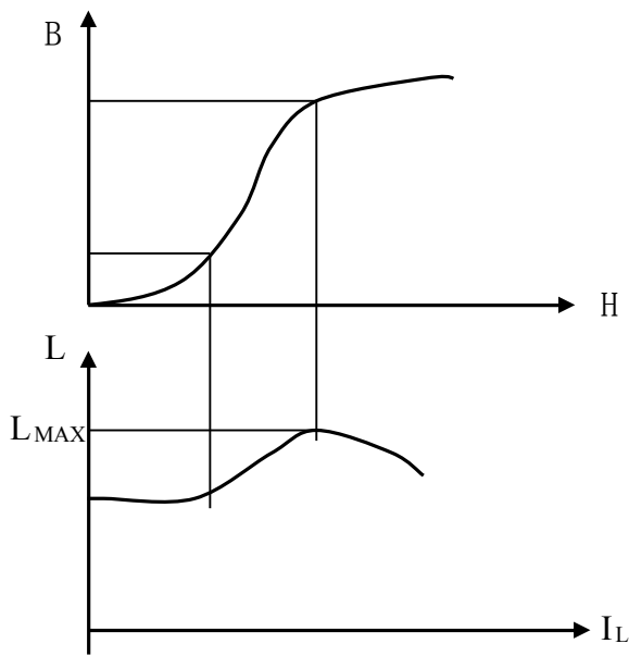
图 3-3 磁场强度、电感量相互关系图
