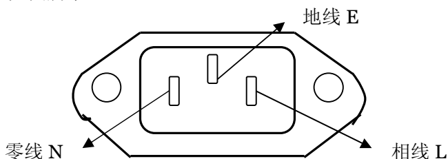
图 3-1 电源插座连接方法（插头的正视图或插座的背视图）
