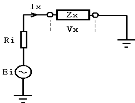
图 2-11 仪器信号源输出等效图
