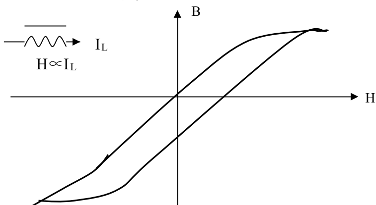
图 3-2 磁芯电感器磁化曲线
