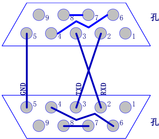
串行通讯电缆连线图
