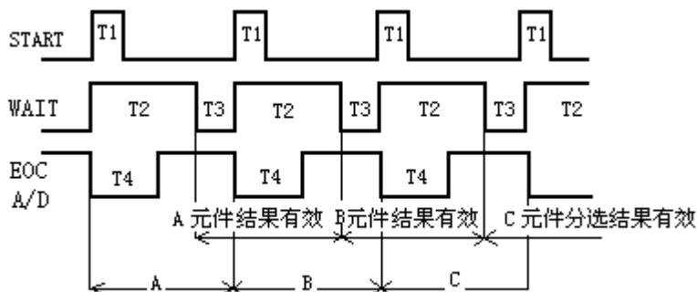
图 2-10 HANDLER 接口工作时序
