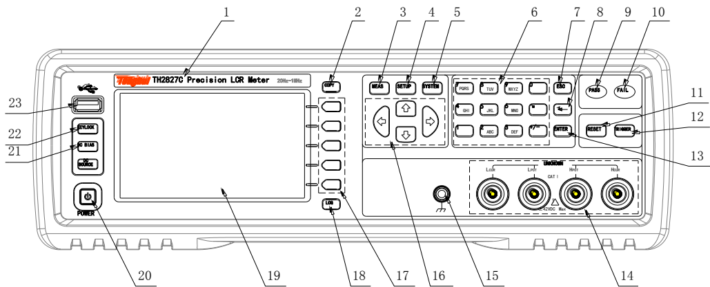
图 2-1. 前面板说明
