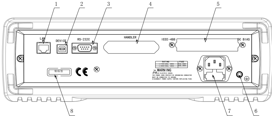
图 2-2. 后面板说明
