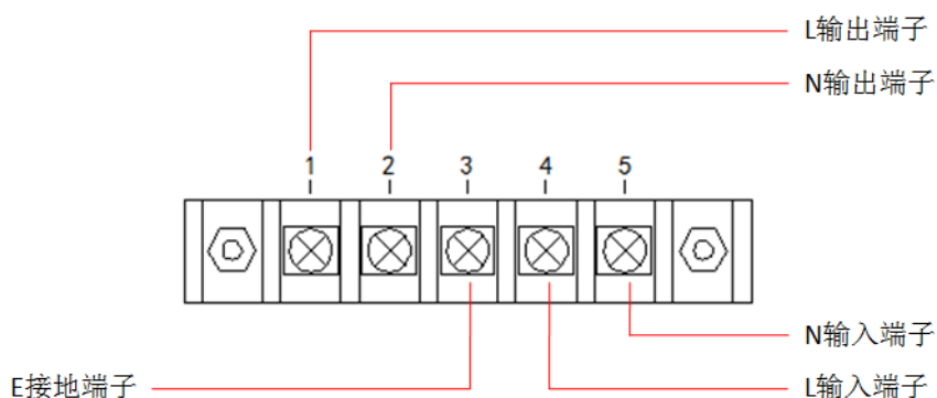
图 1-1 接线示意图
