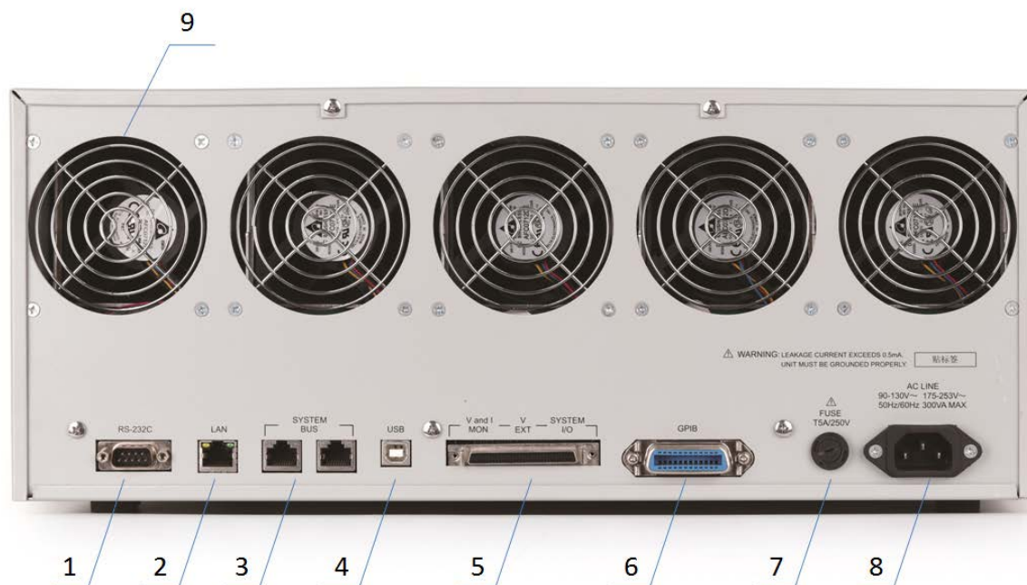
图 2-2 后面板
