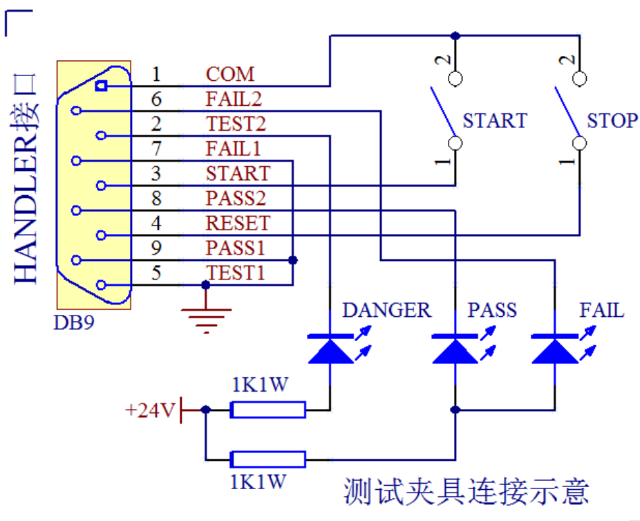
图 4.5.3: HANDLER 外部电路连接示意图（外接电源）
