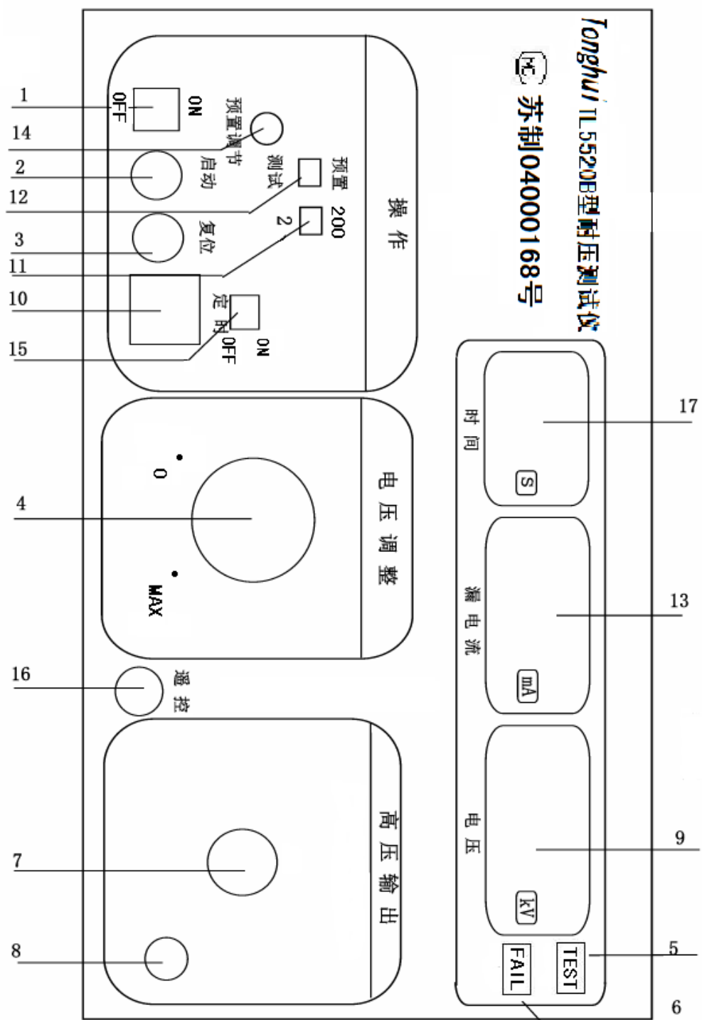
(图二) TL5520B面板示意图
